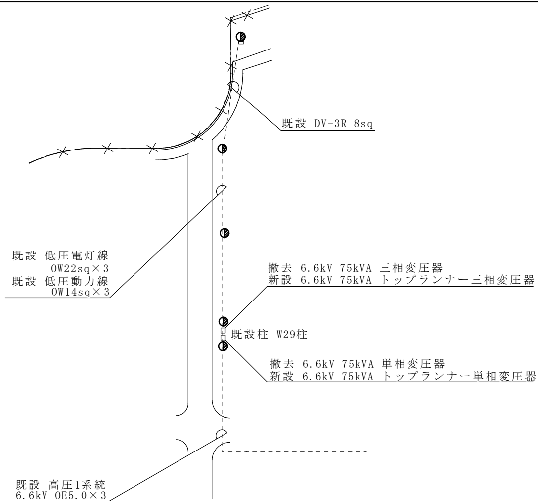
施工箇所① 平面詳細図 S=1/X
