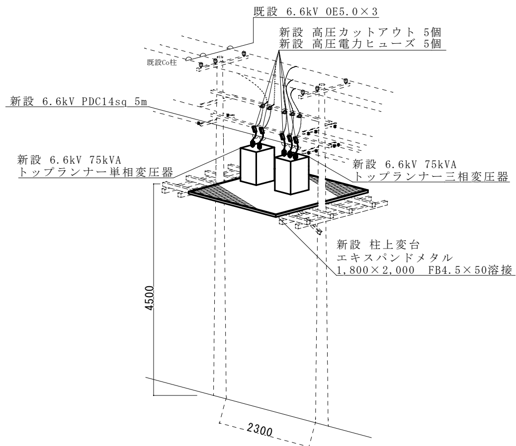
改修後W29柱詳細標準図 S=1/X
