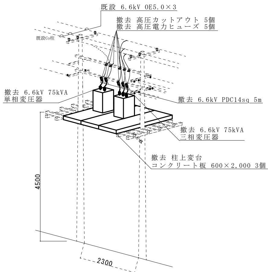
既設 W29 柱詳細標準図 S = 1/X
