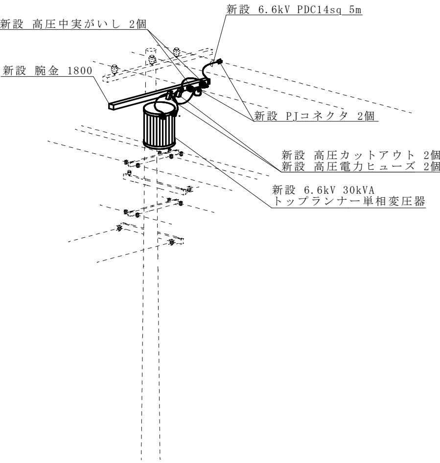
改修後W21柱詳細標準図 S=1/X
