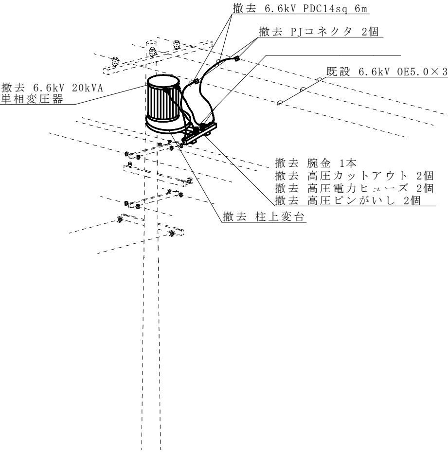
既設W21柱詳細標準図 S=1/X
