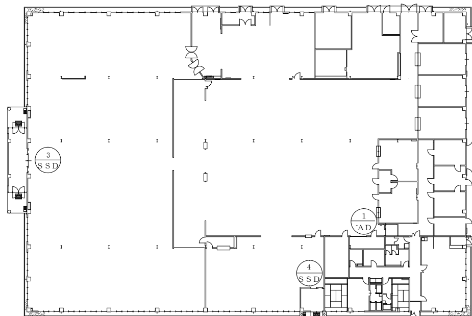
218号建物平面図 S=1/400
