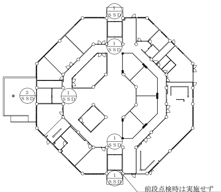
190号建物平面図 S=1/400
