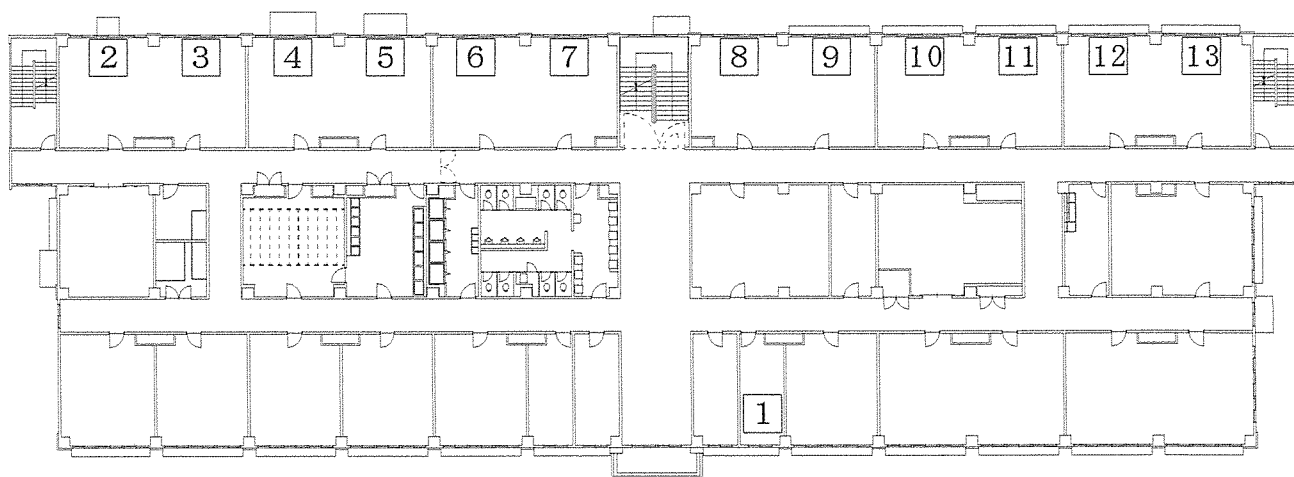
2 階平面図
