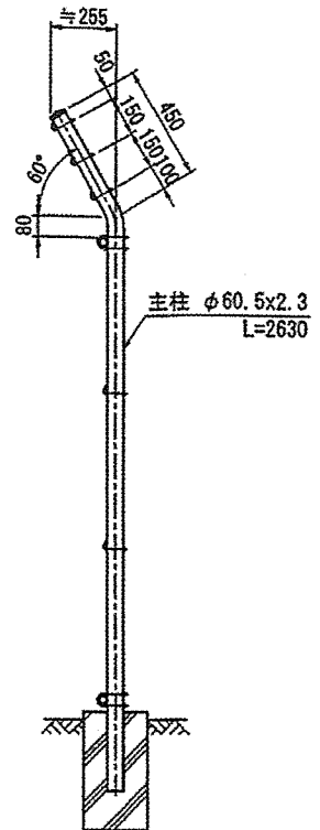
側面図 (S=1/30)
