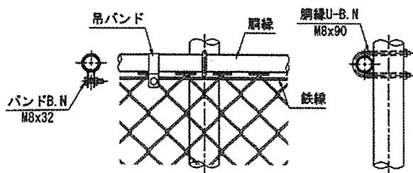
帯縁取付詳細
