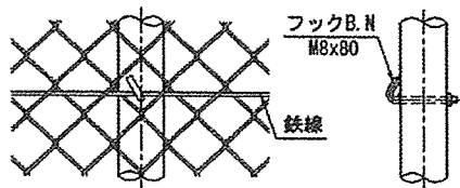
鉄線取付詳細
