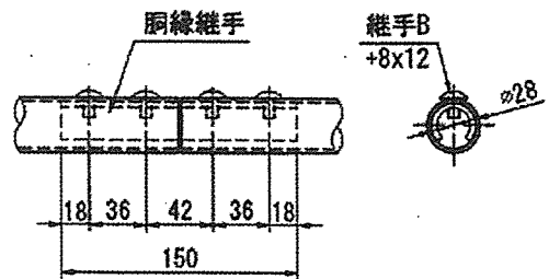
帯縁継手取付詳細
