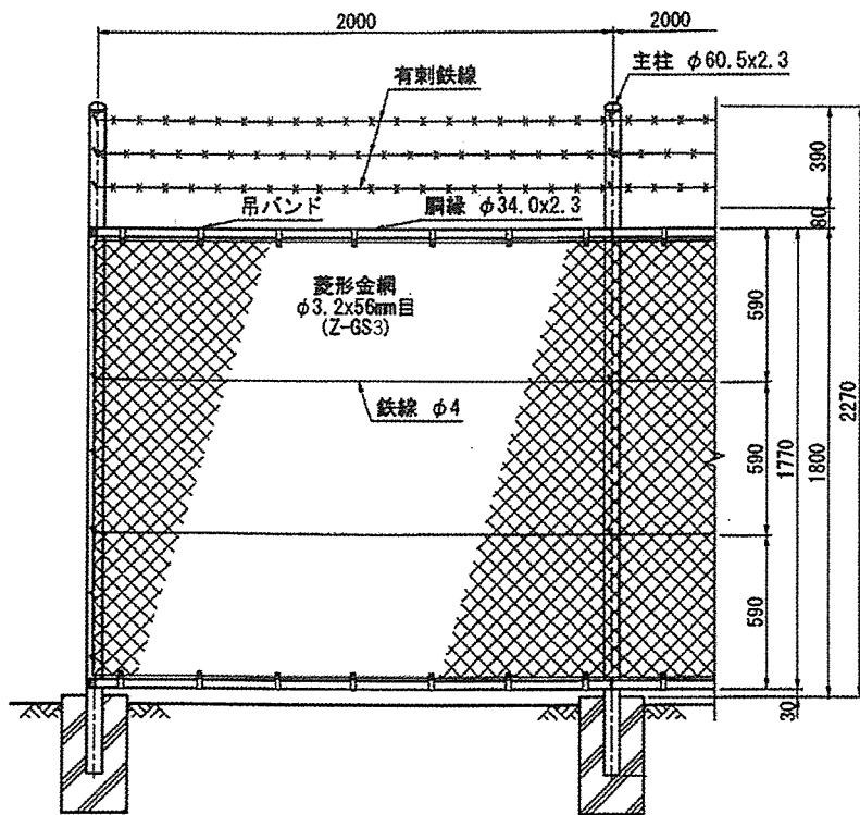
付図 1-外観、形状及び寸法
