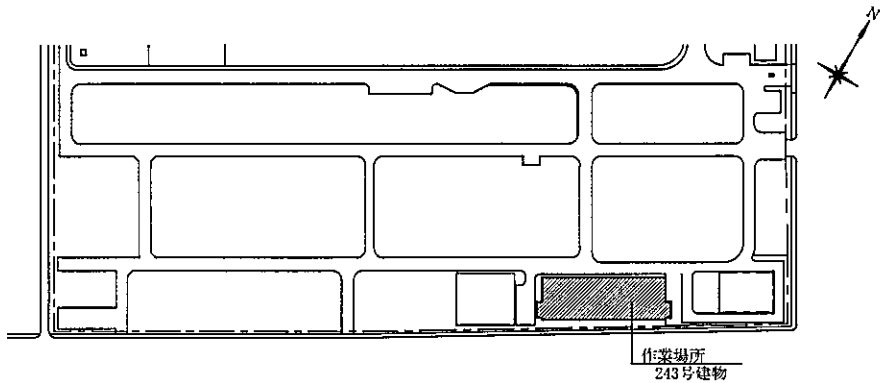
配置図 S=1/3,000
