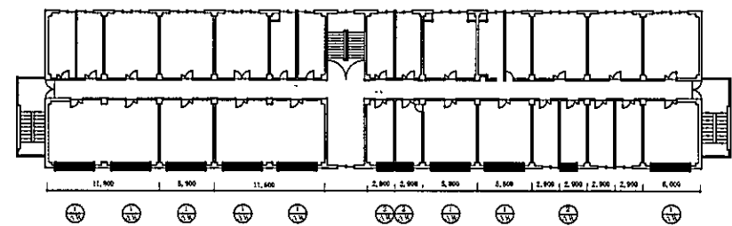
243号建物3F平面図 (2重窓設置・ブラインド用金具設置)
