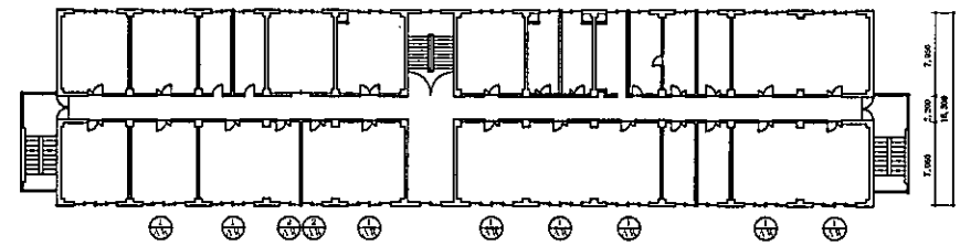
243号建物2F平面図 (ブラインド用金具設置)
