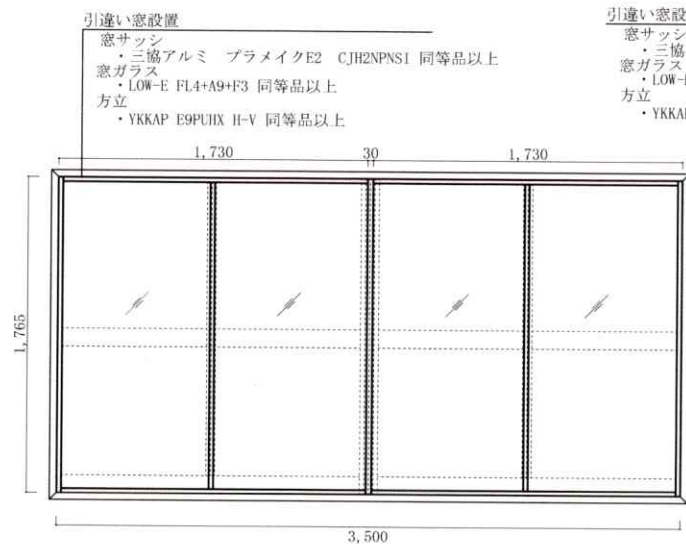
施工詳細図 (AW1)
