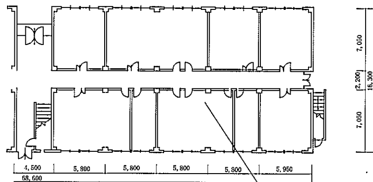
171号平面図
