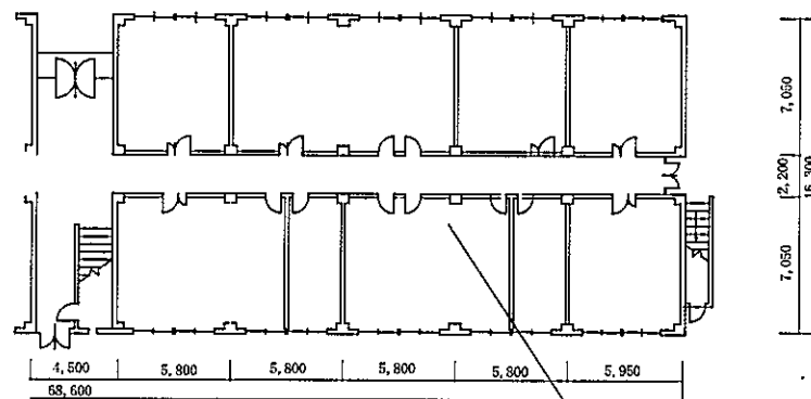
171号平面図
