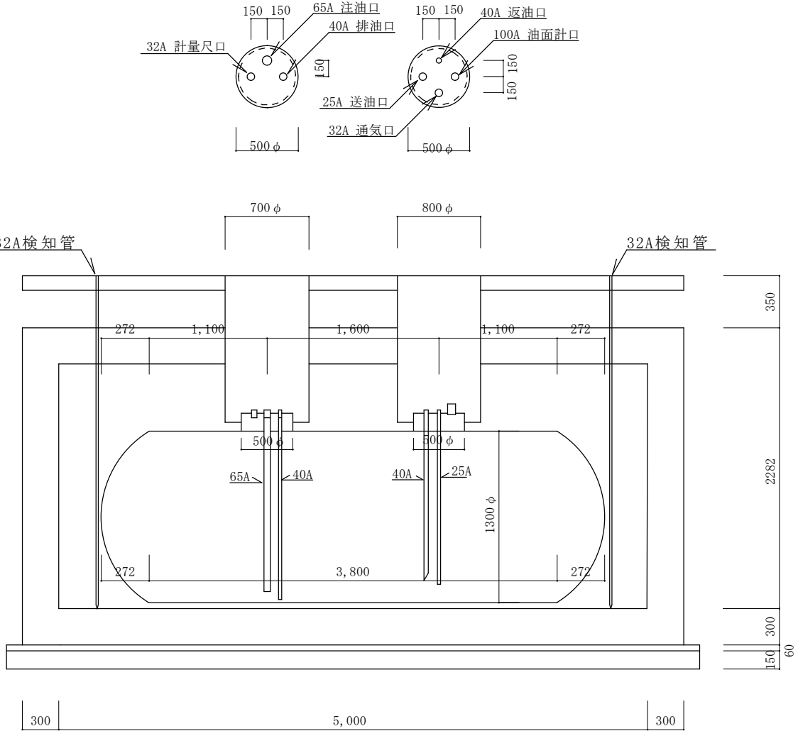
本宮山無線中継所 地下タンク埋設図 1 / X
