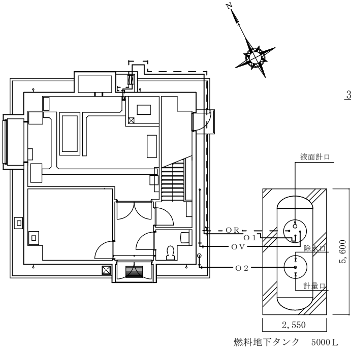
本宮山無線中継所 1 階平面図 1 / X
