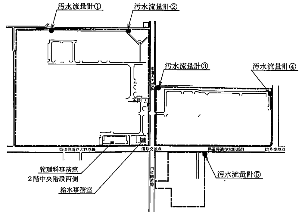
駐屯地配置図 S = 1/5,000
