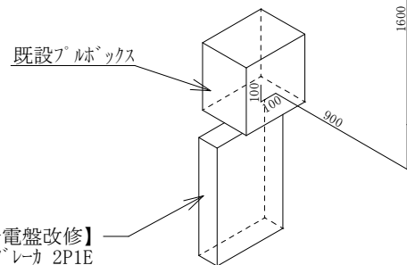
アイソメ図 S=1/40
