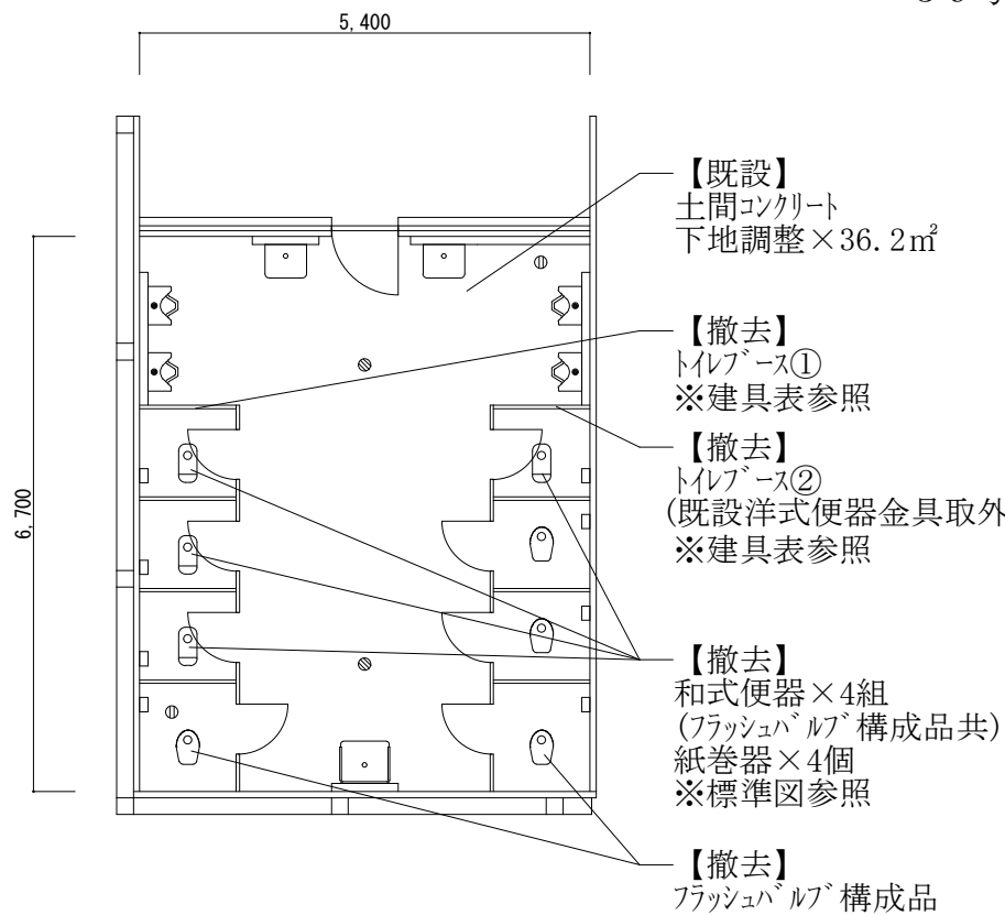
施工場所詳細図 (改修前) S=1/100
