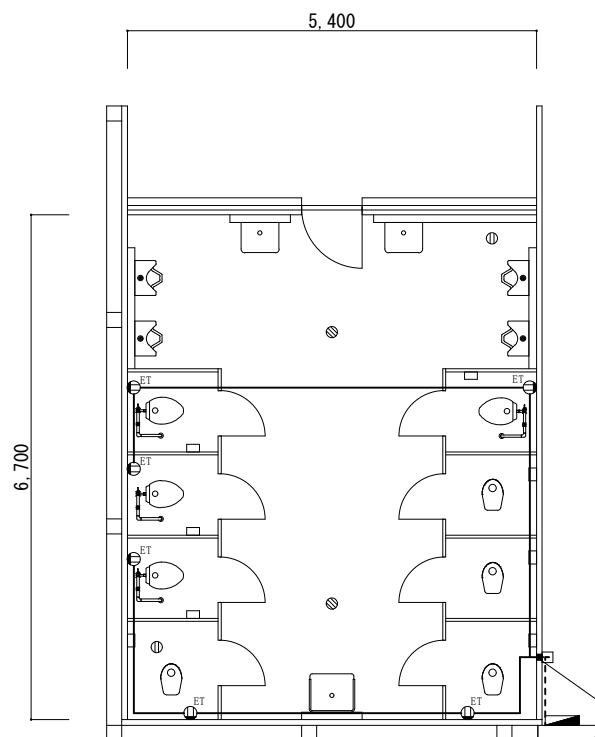
電気設備平面図（改修後） S=1/100
