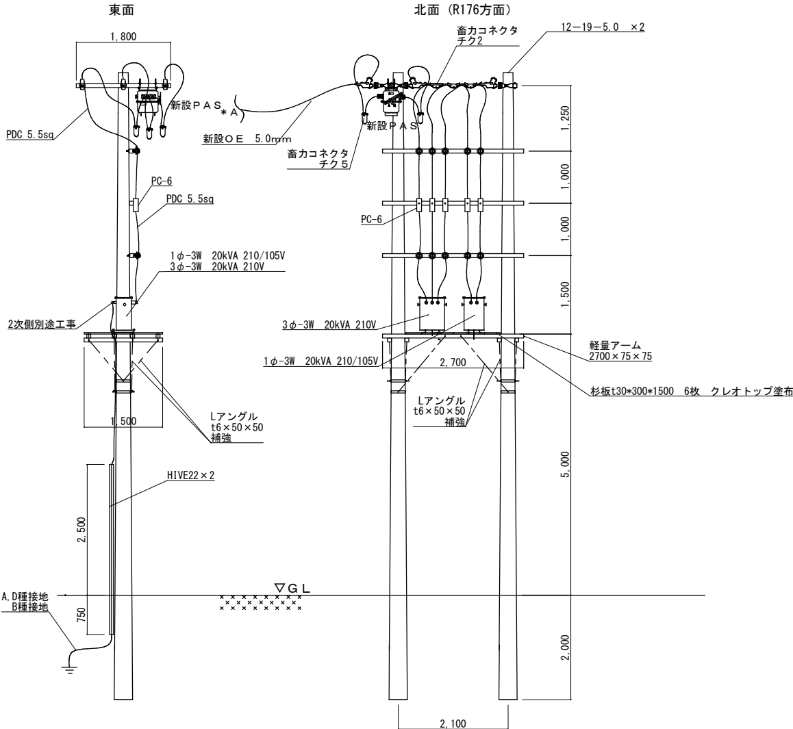
新設32-1号柱分岐柱上変台
