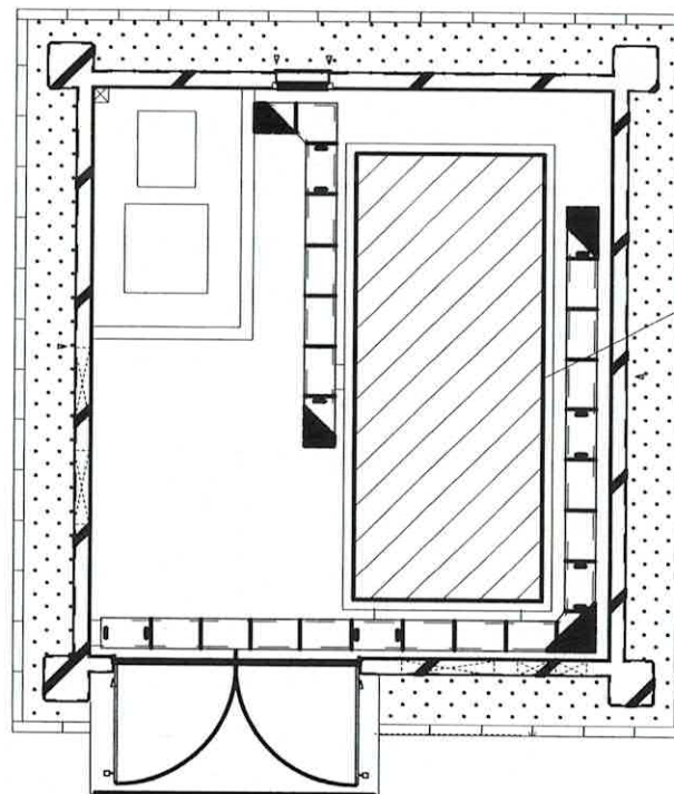
発電機室平面図 S=1/100
