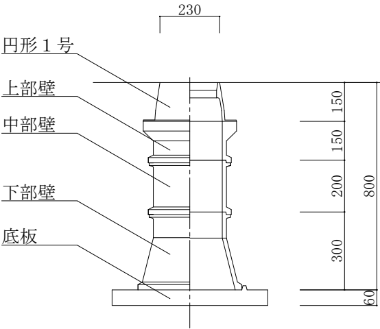
仕切弁筐標準図 (150A) S = 1/20
