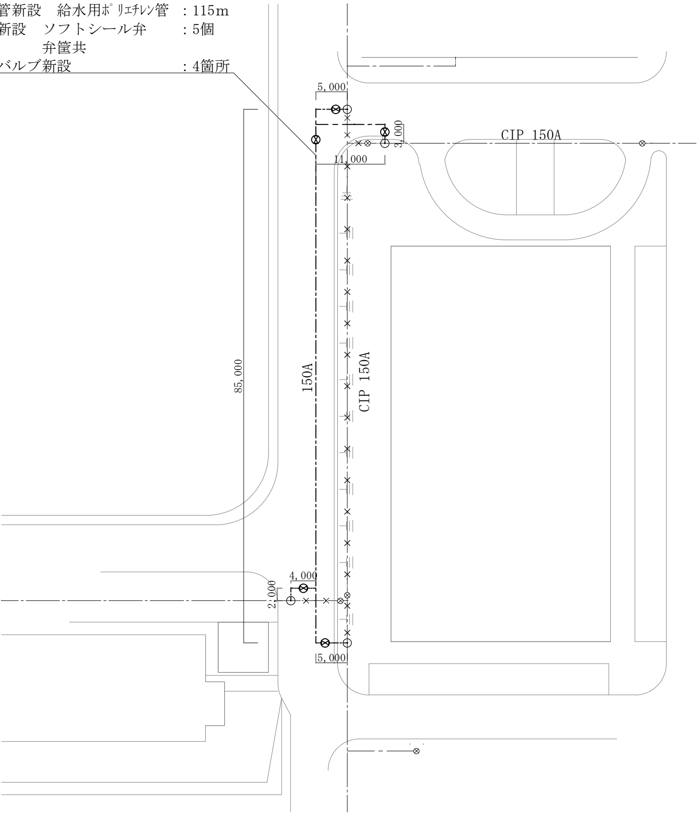
改修給水配管図 S = 1/600
