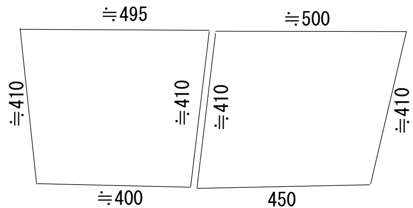
【既設】側溝蓋平面図
