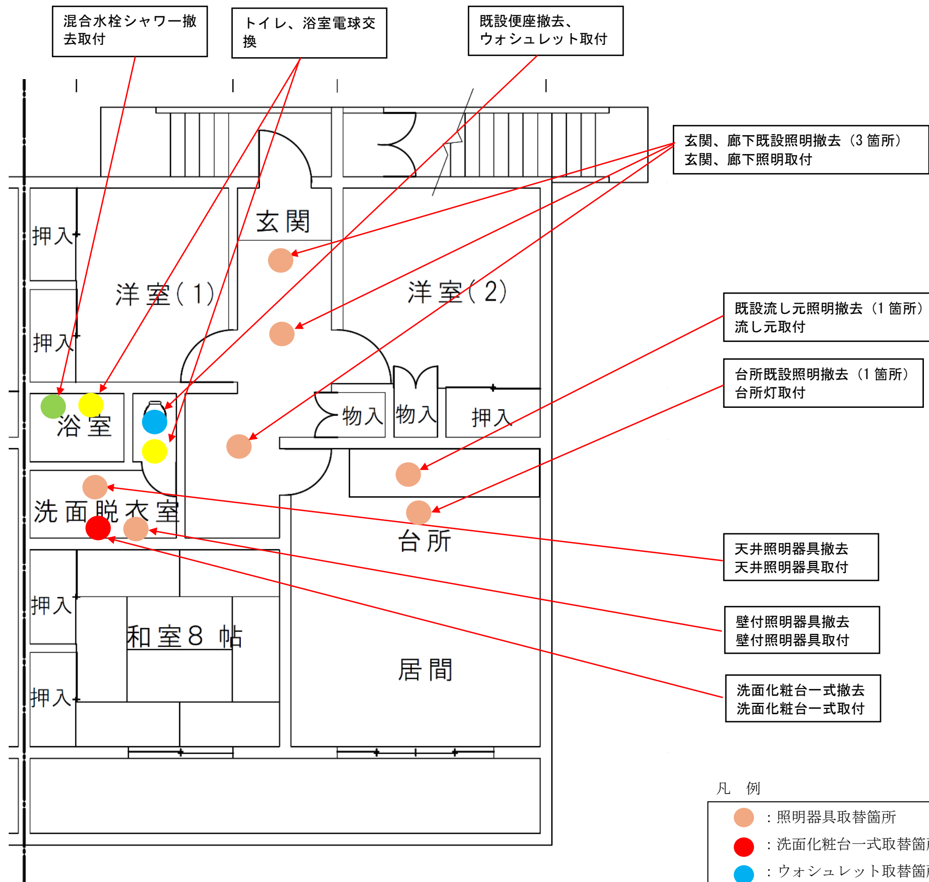
野畑宿舎2号棟平面図
