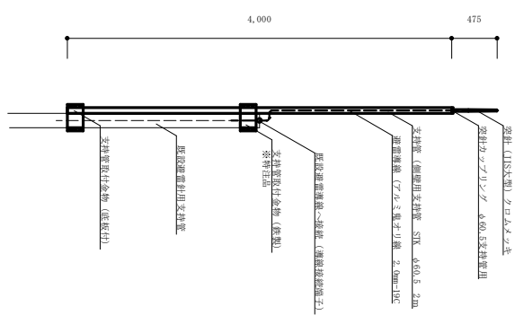
避雷針設置詳細図 S=1/50
