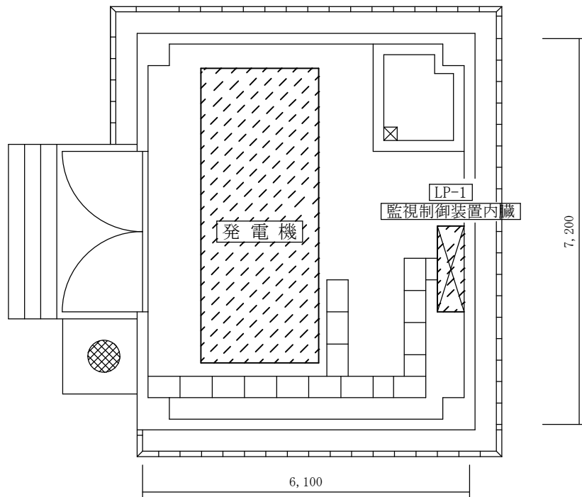
172号建物平面図 S = 1/100
