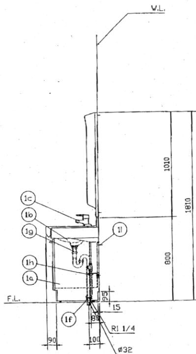
既設洗面化粧台図 (105～510 (30戸)) S=1/X
