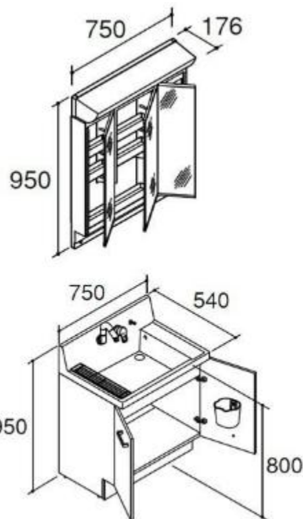
新設洗面化粧台図 (105～510 (30戸)) S=1/X
