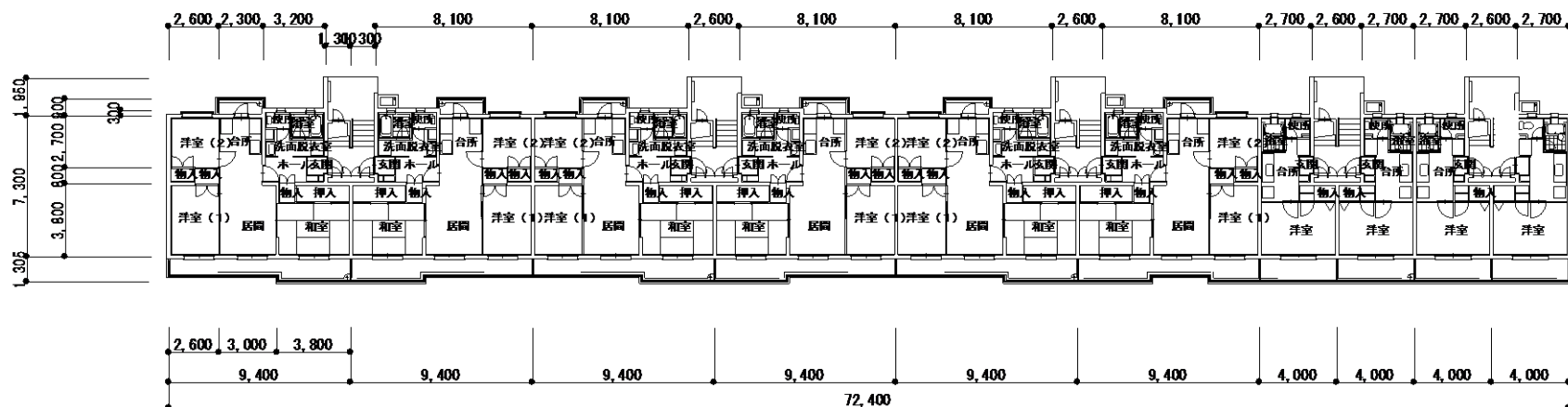
平面図 (1階～5階)
