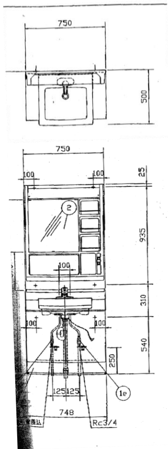
既設洗面化粧台図 (105～510 (30戸)) S=1/X
