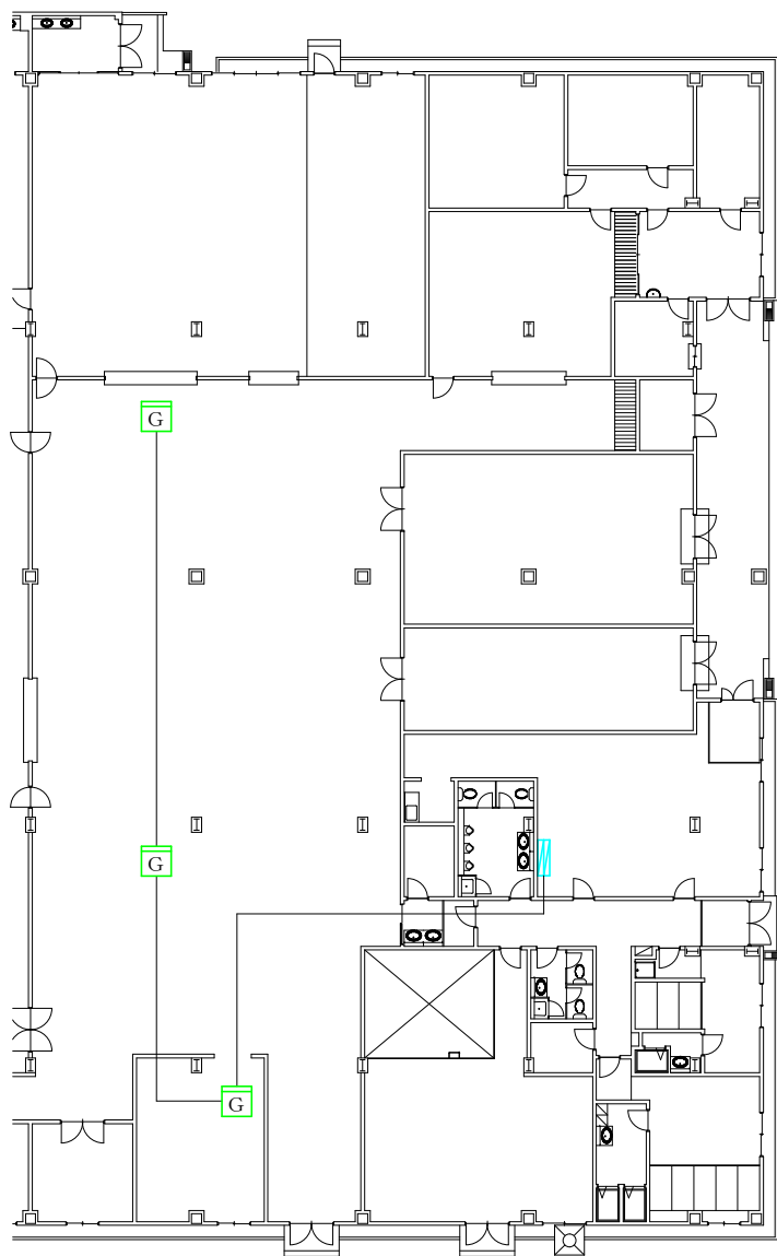
ガス警報器系統図 S=1/400
