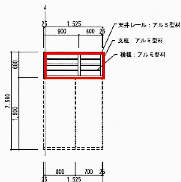
【立 面 図】
