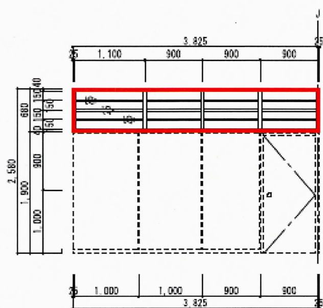
【立 面 図】
