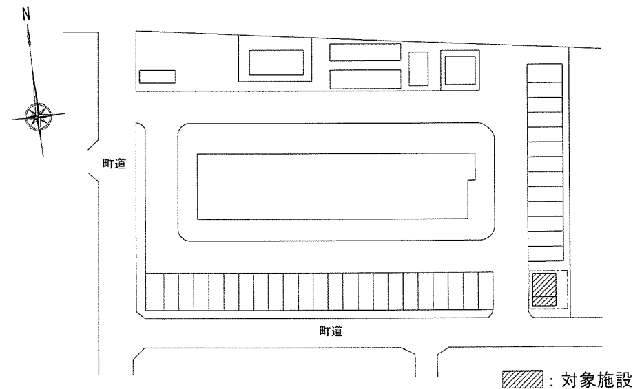
第2赤岡宿舎配置図 S=1/600
