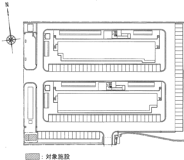
香我美宿舎配置図 S=1/800
