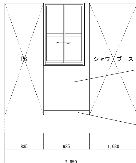
A 展開図 (改修)
