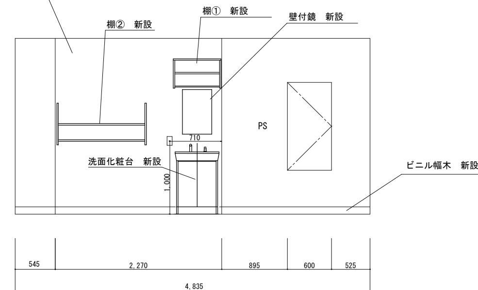
D 展開図 (改修)
