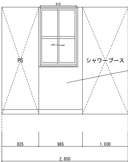
A 展開図（改修）
