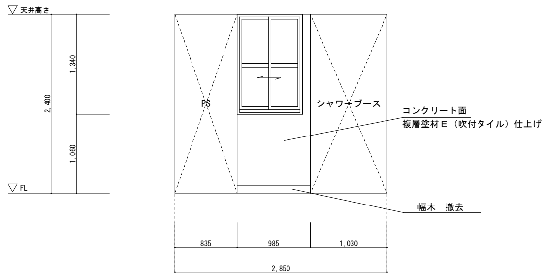
A 展開図（既設）
