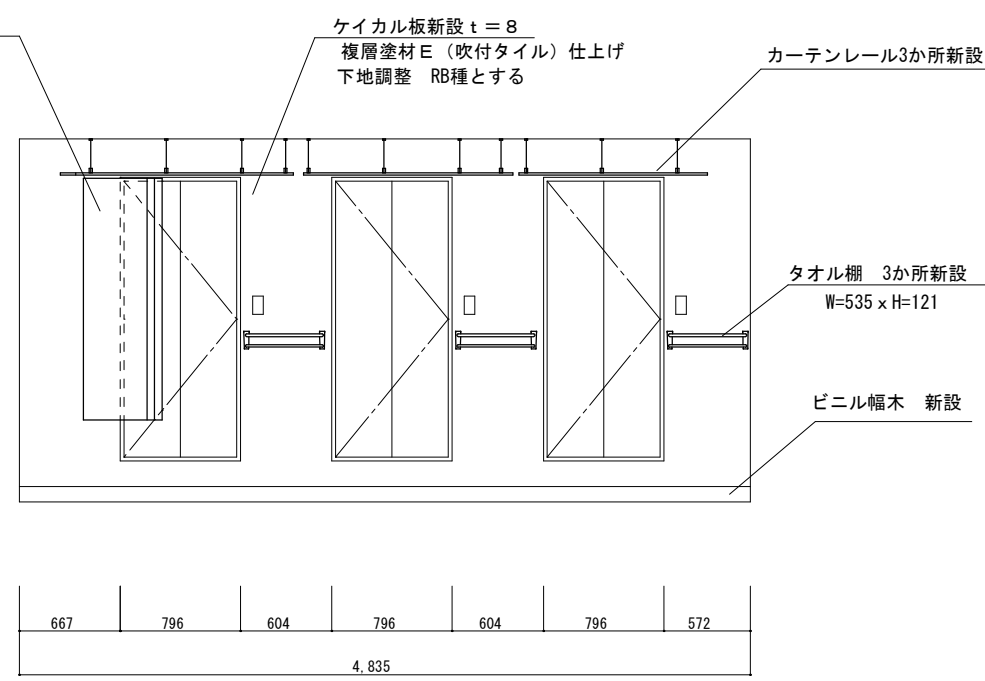
B 展開図 (改修)
