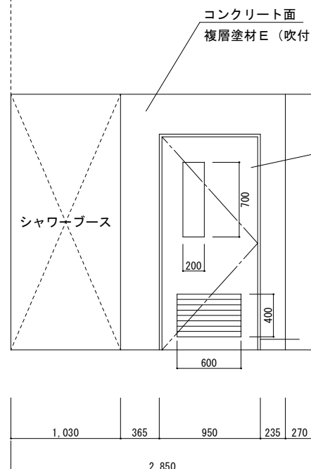
C 展開図 (改修)
