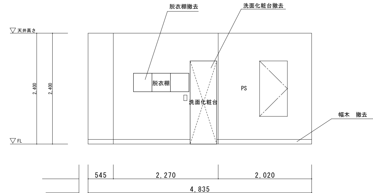
D 展開図（既設）
