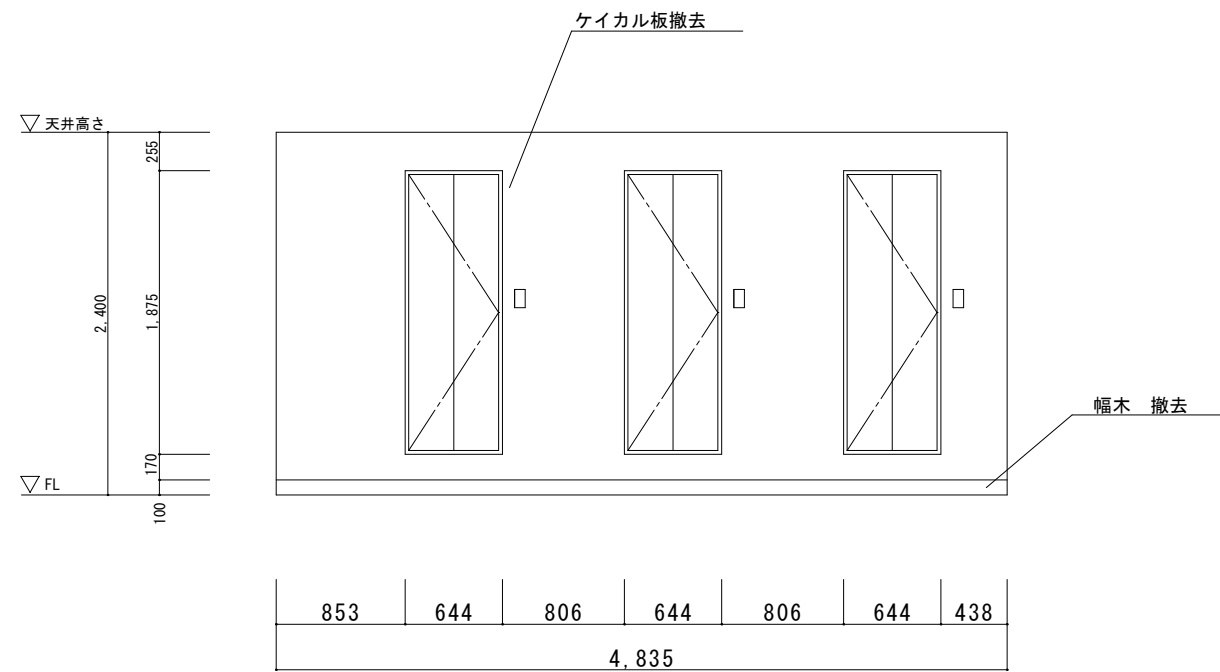
B 展開図（既設）
