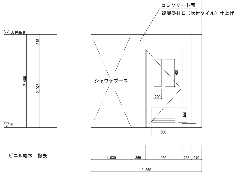
C 展開図（既設）
