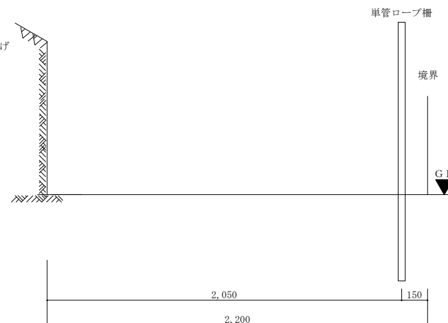
土留鋼板設置断面詳細図(着工前) S:1/15
