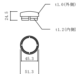
鋼製キャップ S:1/2
