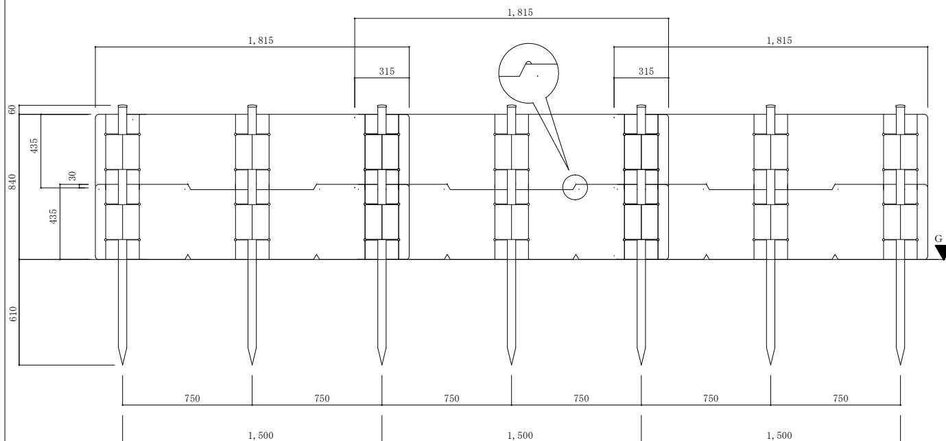
土留鋼板展開図 S:1/15
