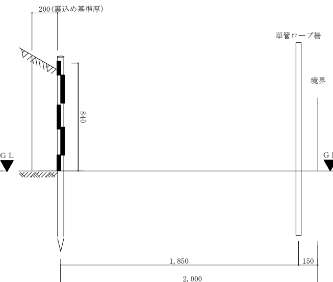
土留鋼板設置断面詳細図(着工後) S:1/15
