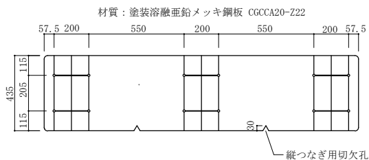
土留鋼板姿図 S:1/15
