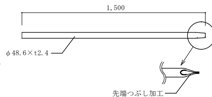
鋼管支柱姿図 S:1/15
