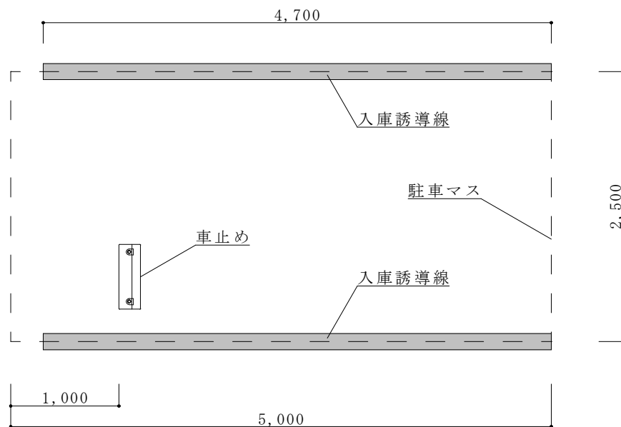
駐車場標準平面図 S=1/50
