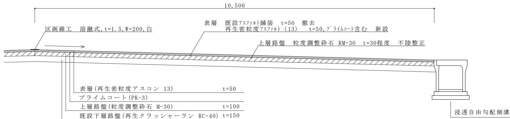
舗装工 標準断面図 S=1/50
