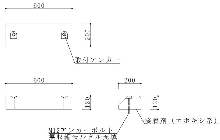
車止め標準図 S=1/20
