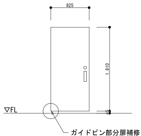
トイレブース扉補修箇所 S=1：50
