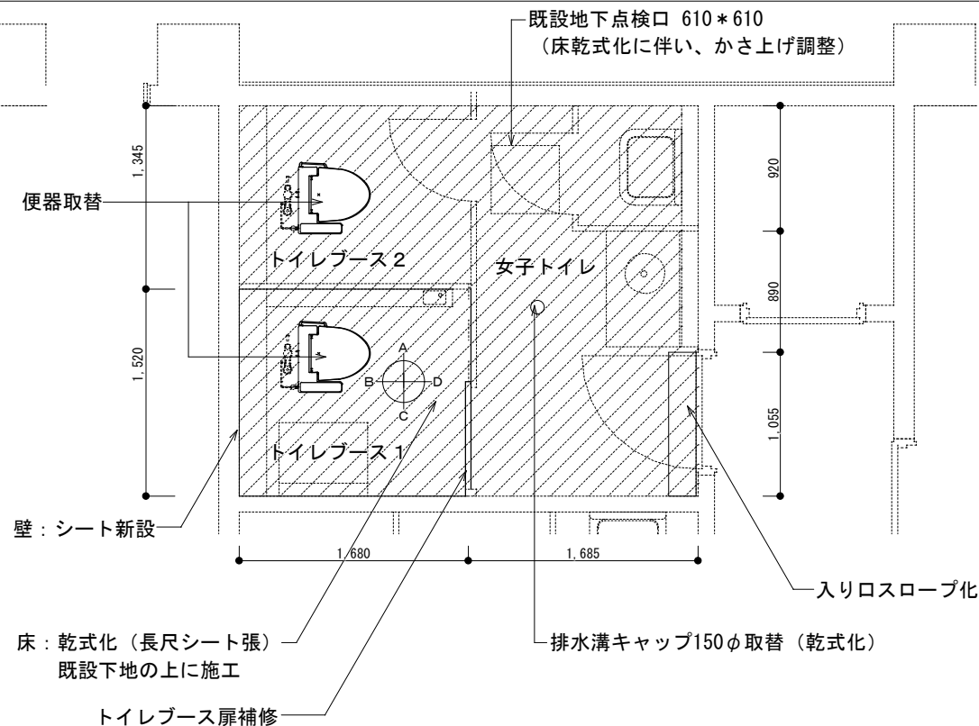
改修後トイレ平面図 S=1:50
