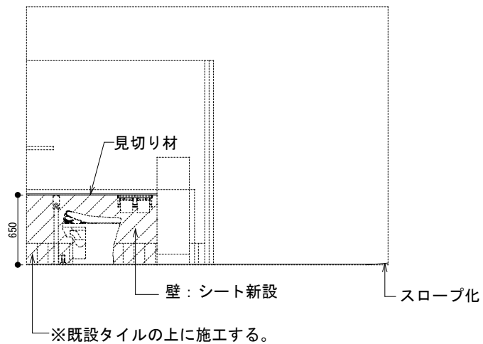
A面展開図図 S=1：50
