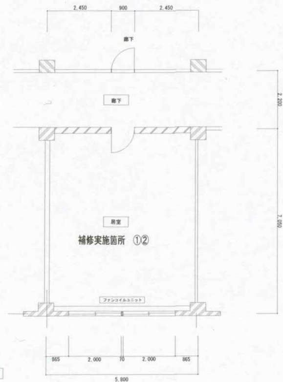
補修居室標準既設平面図
