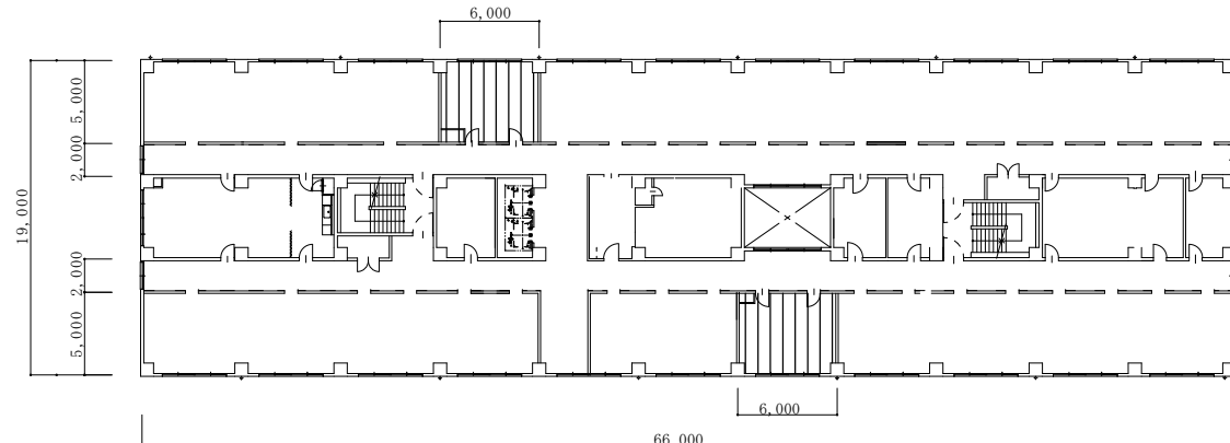
4階平面図
