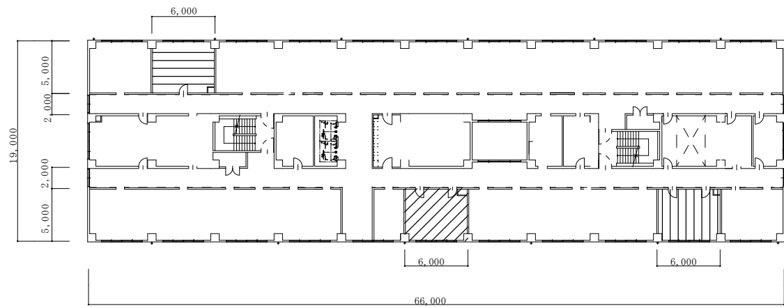
6階平面図
