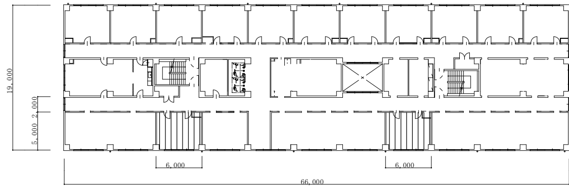
5階平面図
