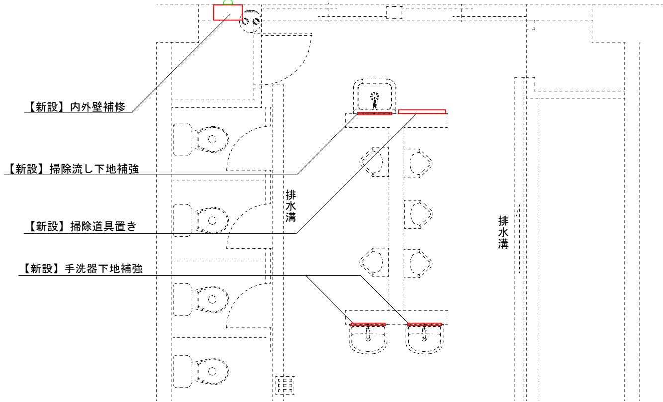
【改修後】3階 男性トイレ 建築平面図
