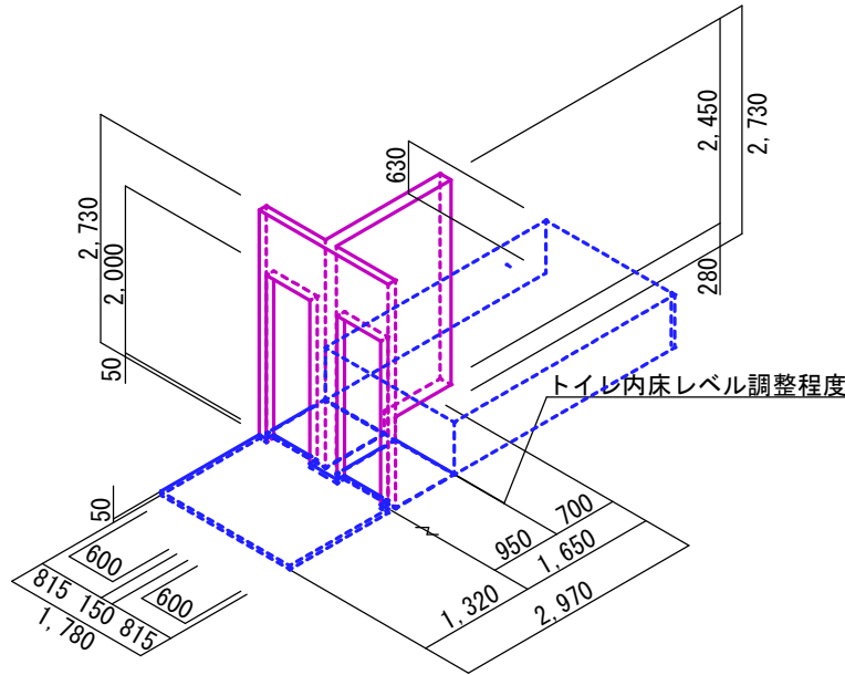
【新設】通路女性トイレ 間仕切り壁・床・天井等 視点B透視図
