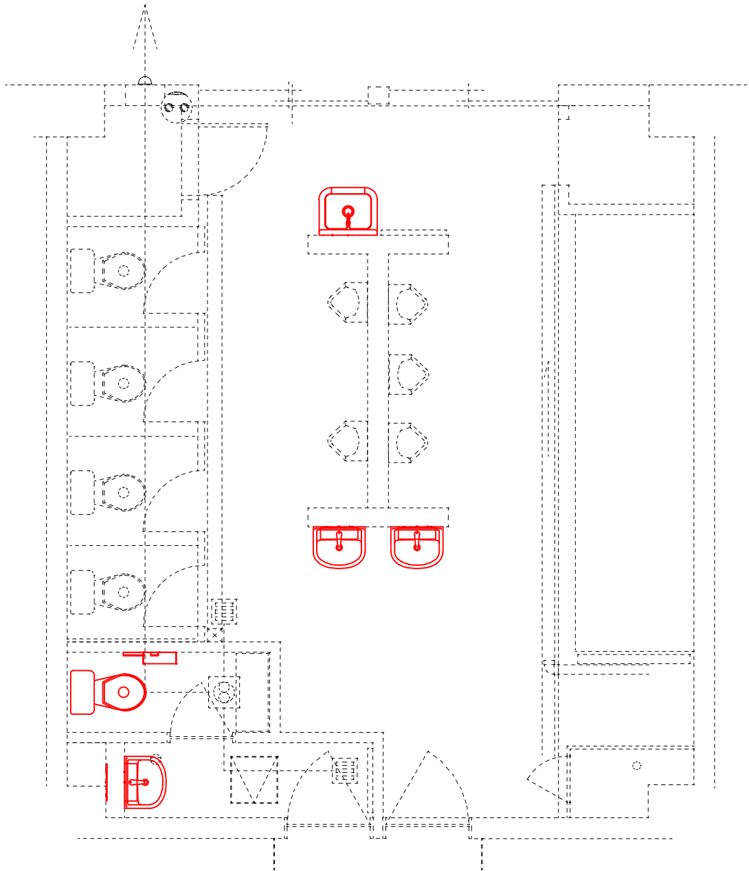
【改修後】給水管工事 女性トイレ他 平面図
