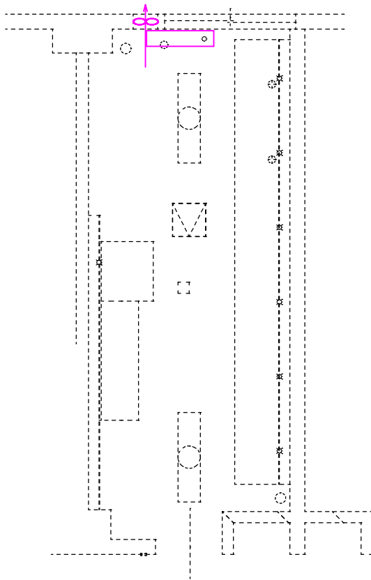
【改修前】機械設備工事 1F平面図
