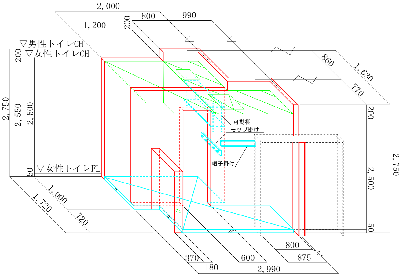
【新設】間仕切り壁・床・天井 視点A透視図
