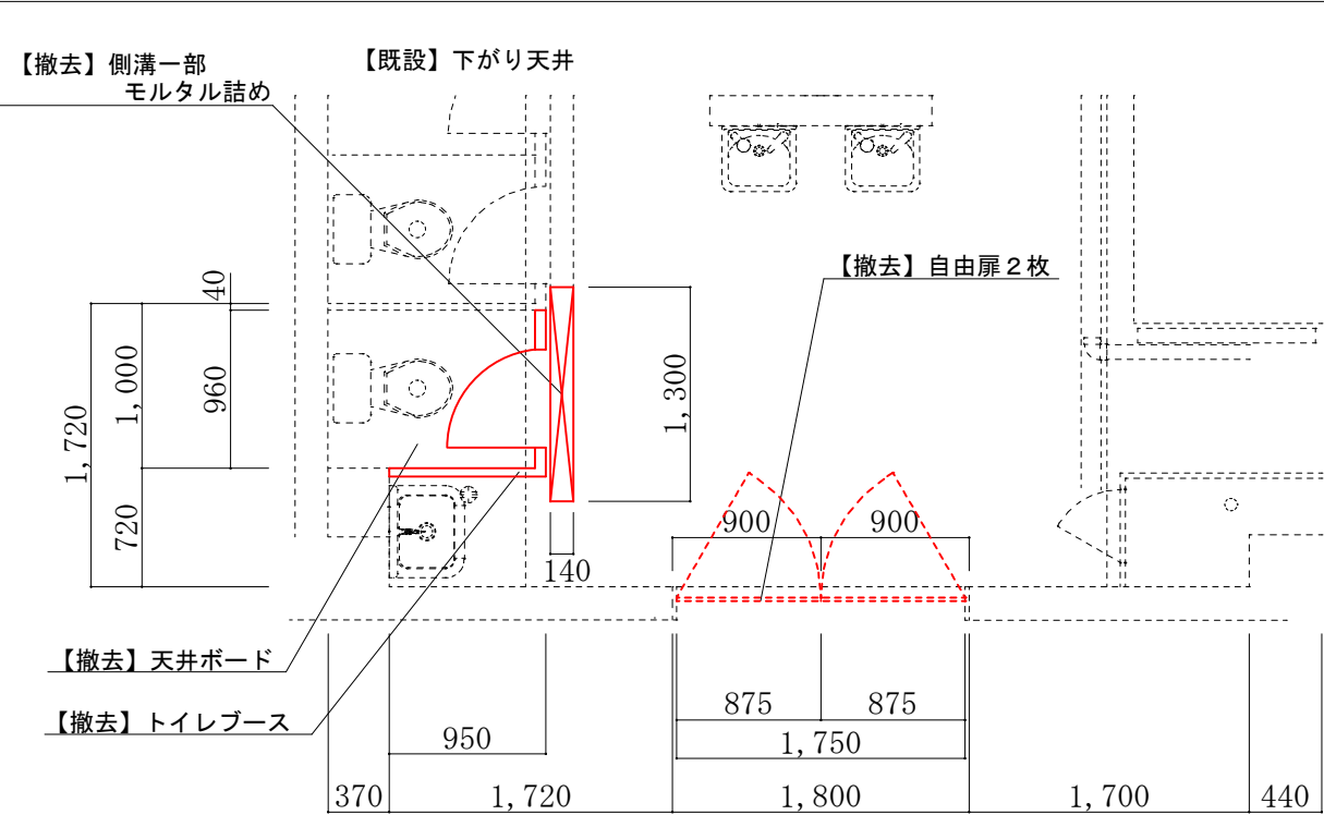
【改修前】女性トイレ 建築平面図
