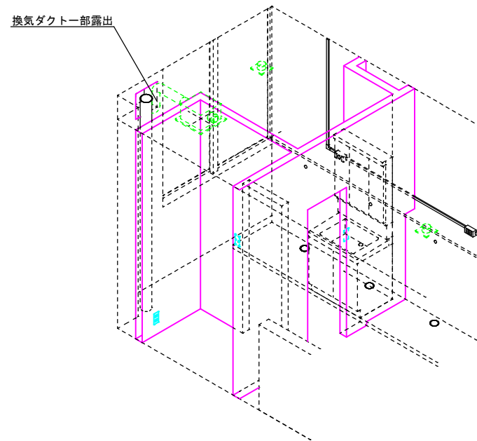
【改修後】 女性トイレ・洗面所透視図
