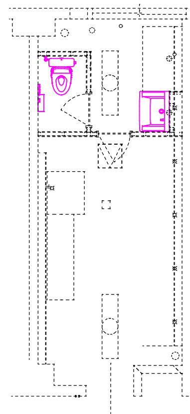
【改修後】衛生設備工事 女性トイレ平面図
