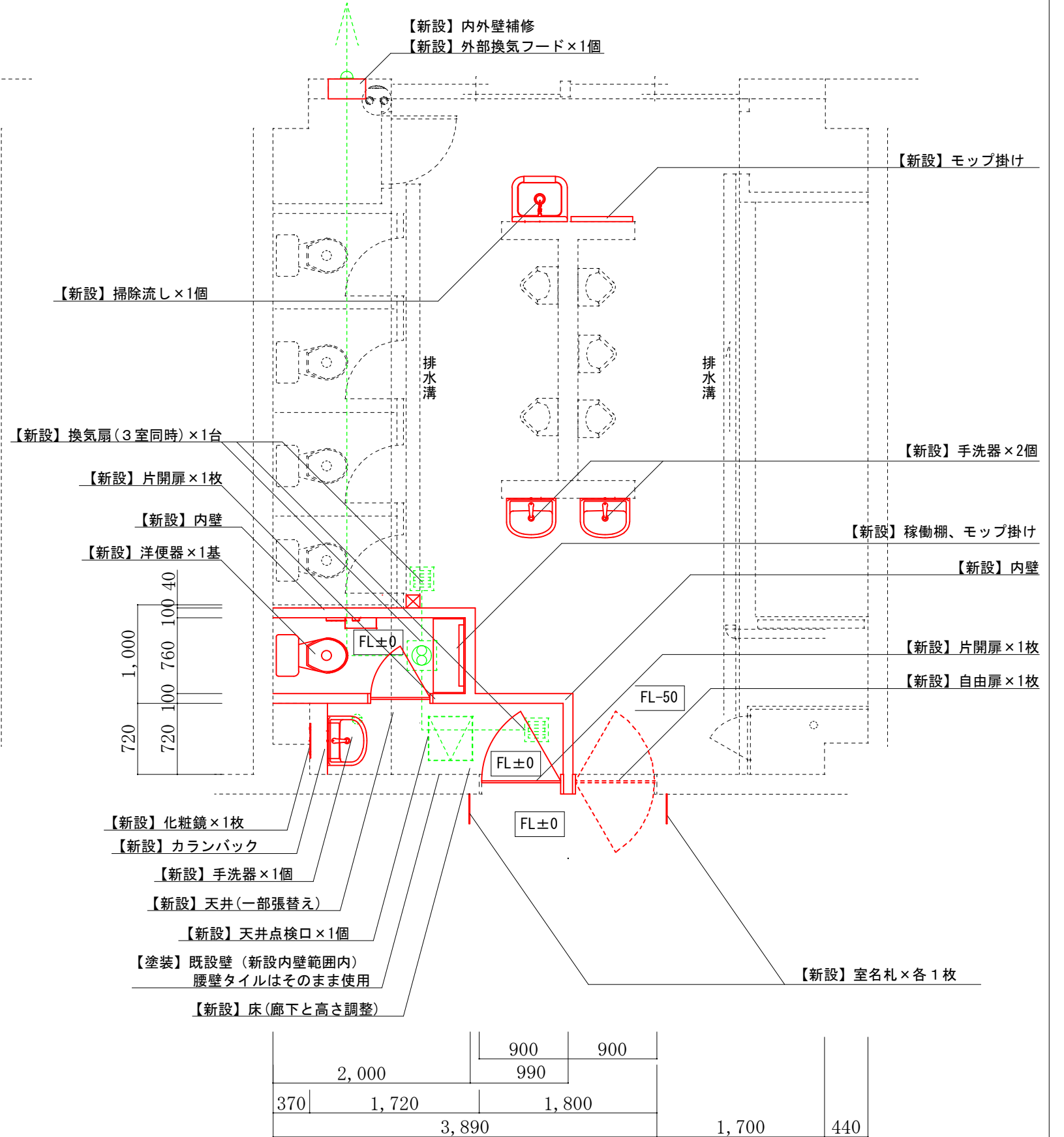
【改修後】概略図
