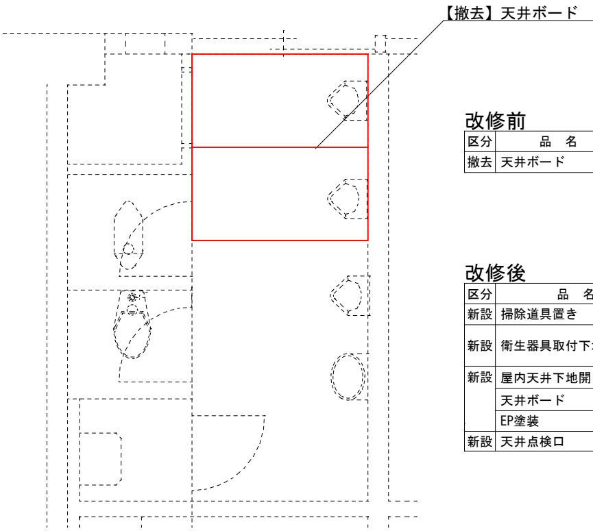
【改修前】2階 男性トイレ 建築平面図
