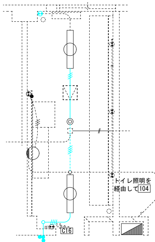
【改修前】電気配線工事 1F平面図
