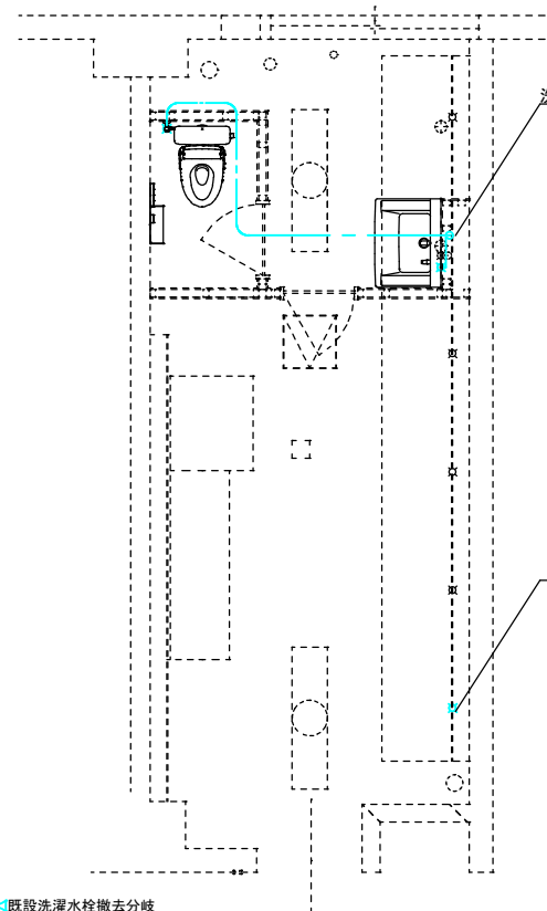
【改修後】給水管工事 女性トイレ平面図
