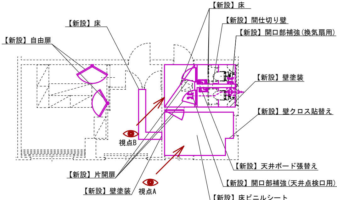
【改修後】1階建築平面図
