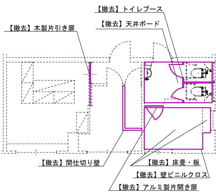
【改修前】1階建築平面図
