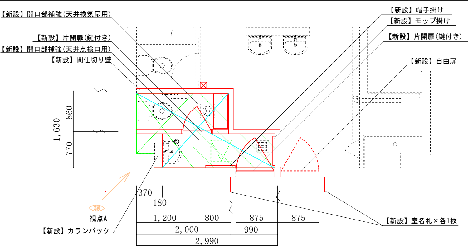
【改修後】女性トイレ建築平面図
