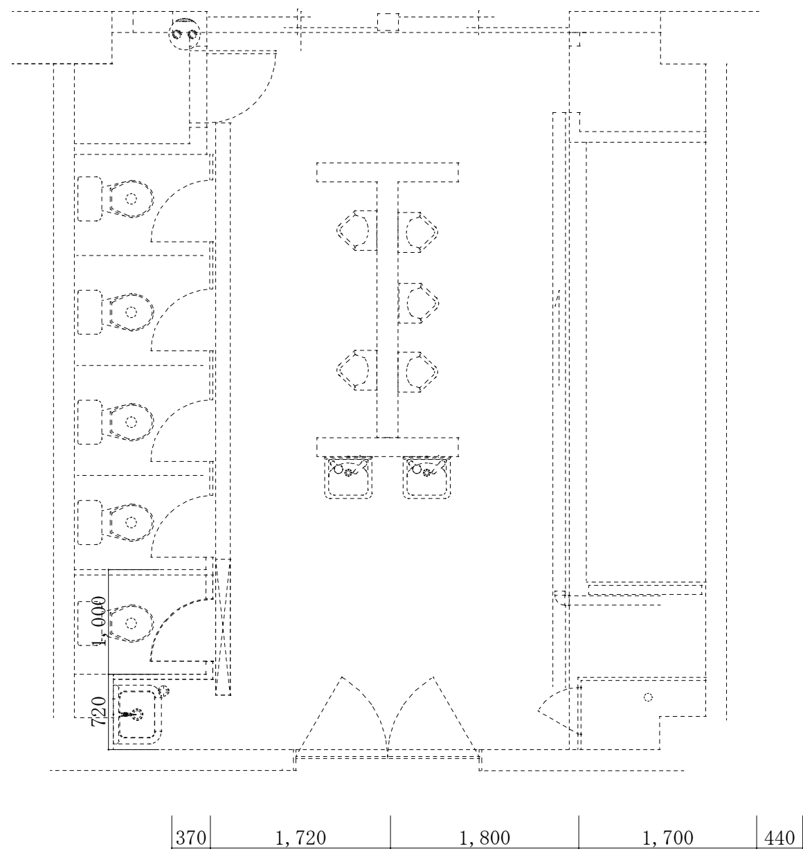
【改修前】機械設備工事 3F平面図
