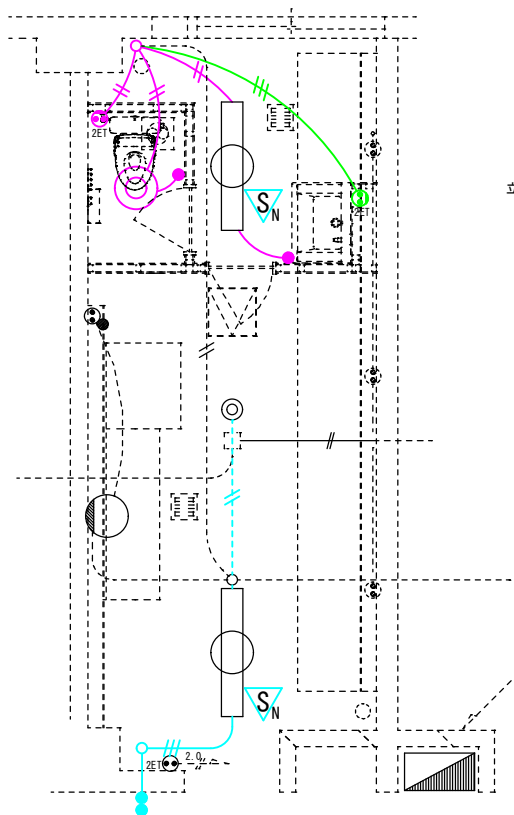
【改修後】電気配線工事 1F平面図
