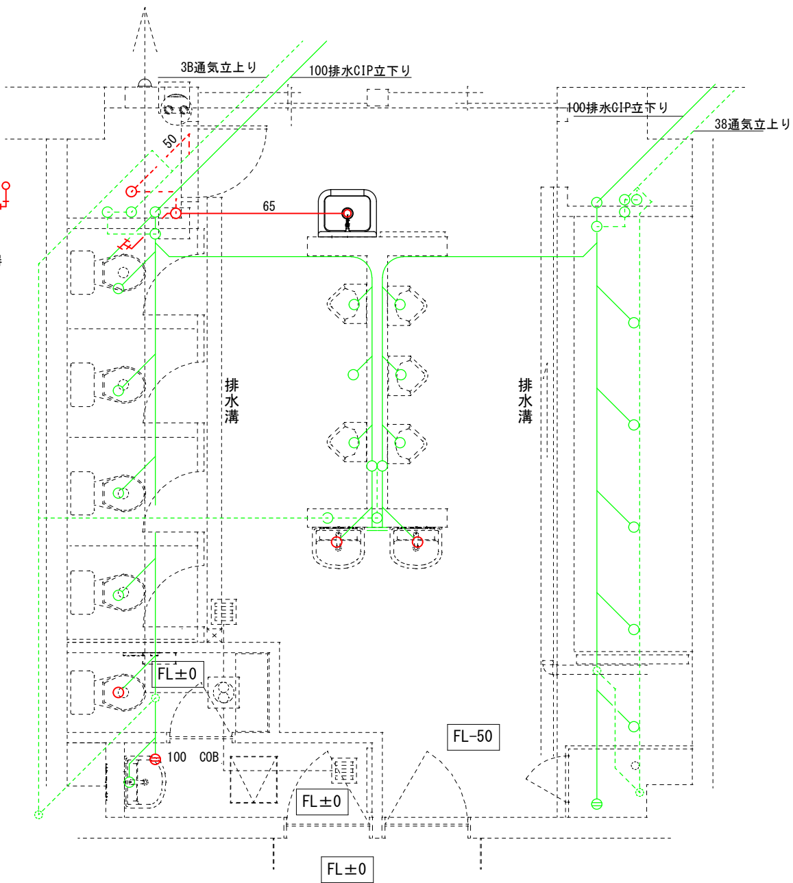
【改修後】排水管工事 女性トイレ平面図
