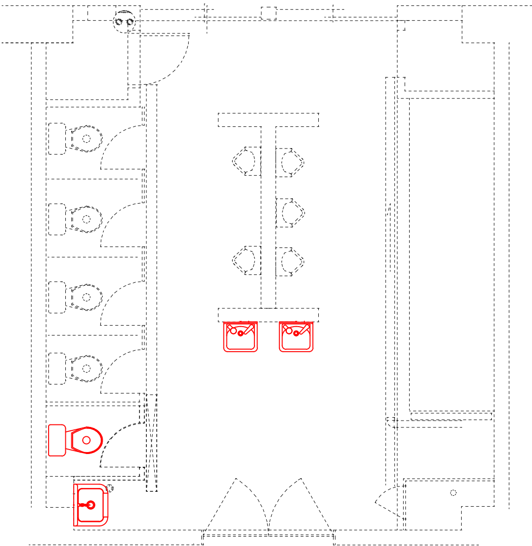
【改修前】給水管工事 女性トイレ他 平面図
