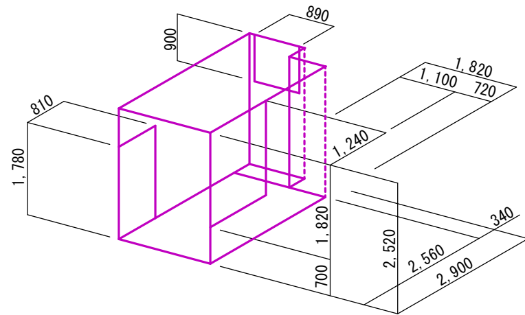
【新設】女性更衣室 壁クロス張替え・床等 視点A透視図
