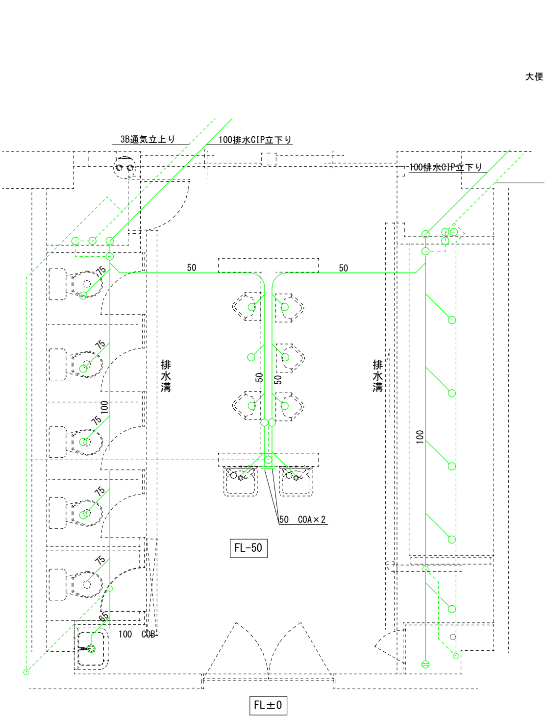
【改修前】排水管工事 女性トイレ平面図
