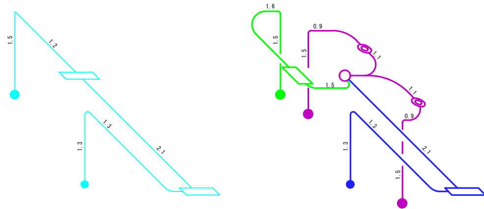
【改修前】照明配線工事 女性トイレ・更衣室
