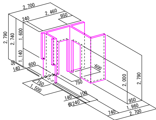
【新設】間仕切り壁 視点A透视图
