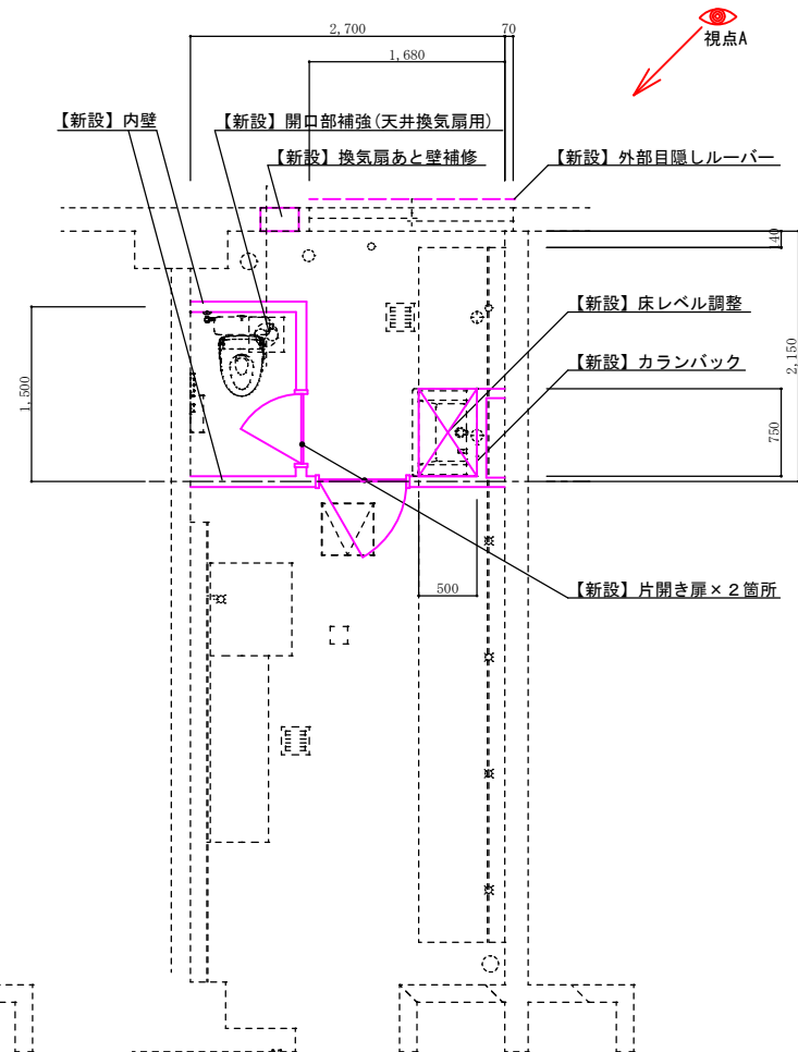
【改修後】女性トイレ・洗面所建築平面図
