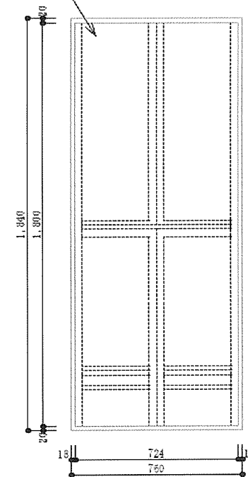
シャワーユニット折戸新設標準図 S=1:20
