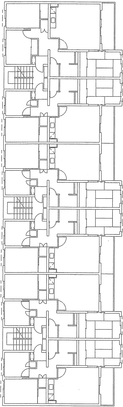
高茶屋第3宿舎A棟1～5階平面図 S=1/X
