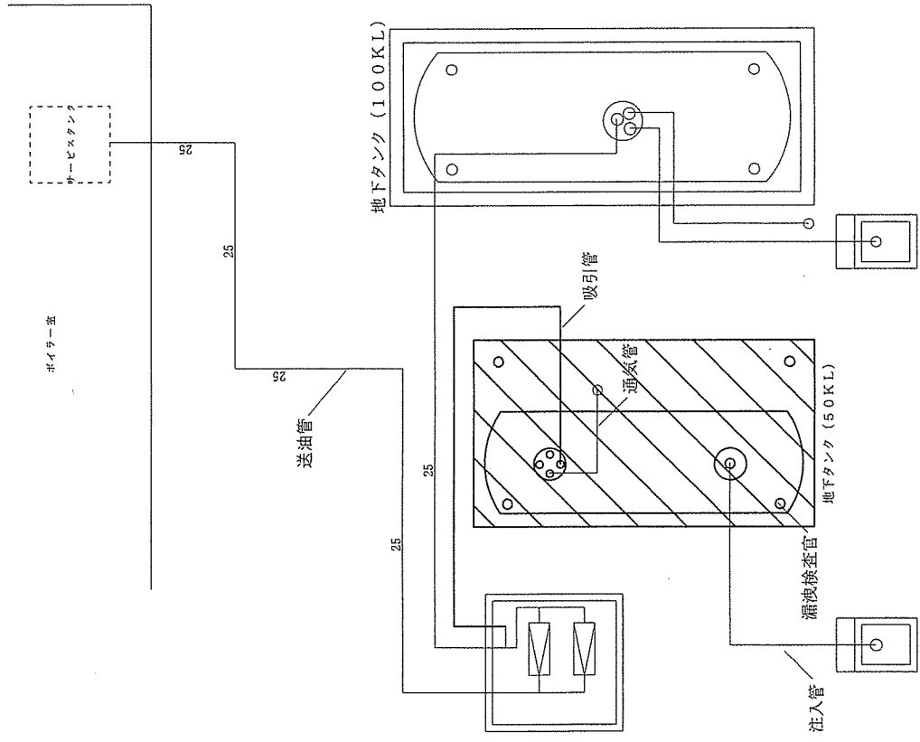
ボイラー用地下タンク等周辺図 S=1/100
