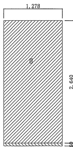
B面施工前 立面図 S=1/50
