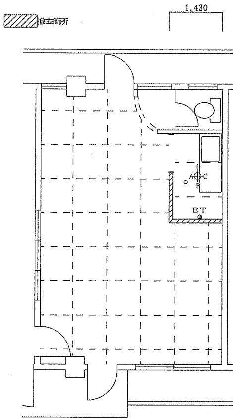
30号建物施工前 平面図 S=1/100
