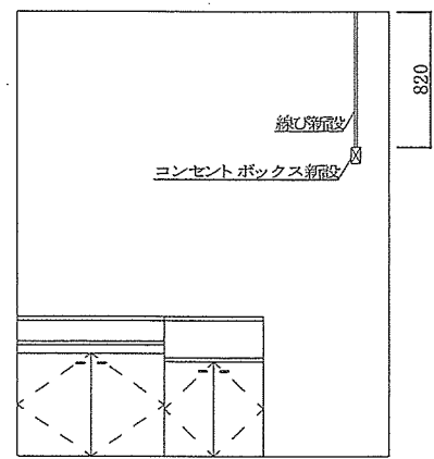
C面施工後 立面図 S=1/50
