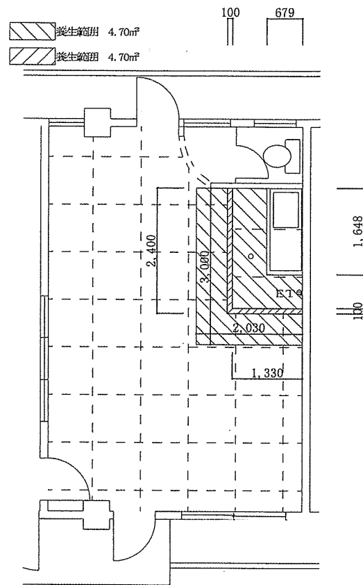
30号建物施工後 平面図 S=1/100
