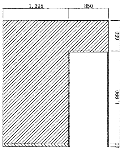
A面施工前 立面図 S=1/50
