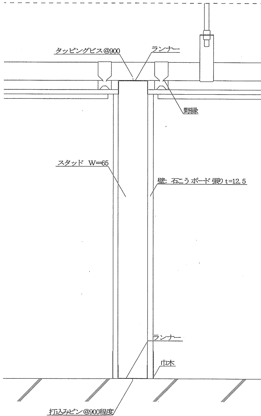
軽量鉄骨間仕切り壁詳細図 S=1/X
