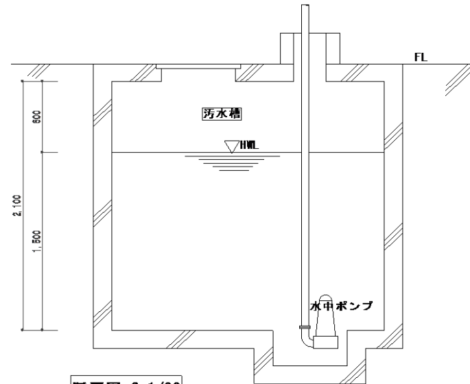
断面図 S=1/30
