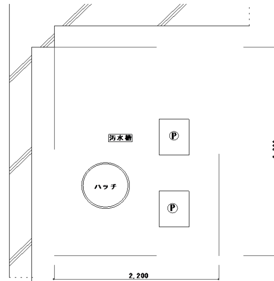
平面図 S=1/30
