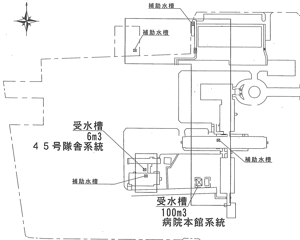
駐屯地配置図 S=1/2,000
