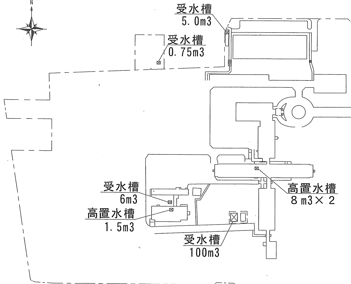
駐屯地配置図 S=1/2,000
