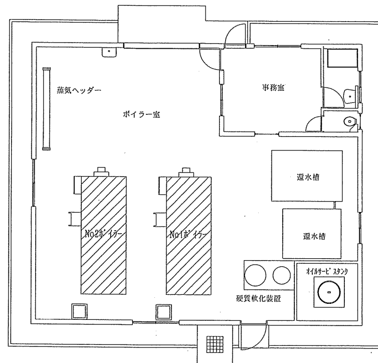
ボイラー室平面図
