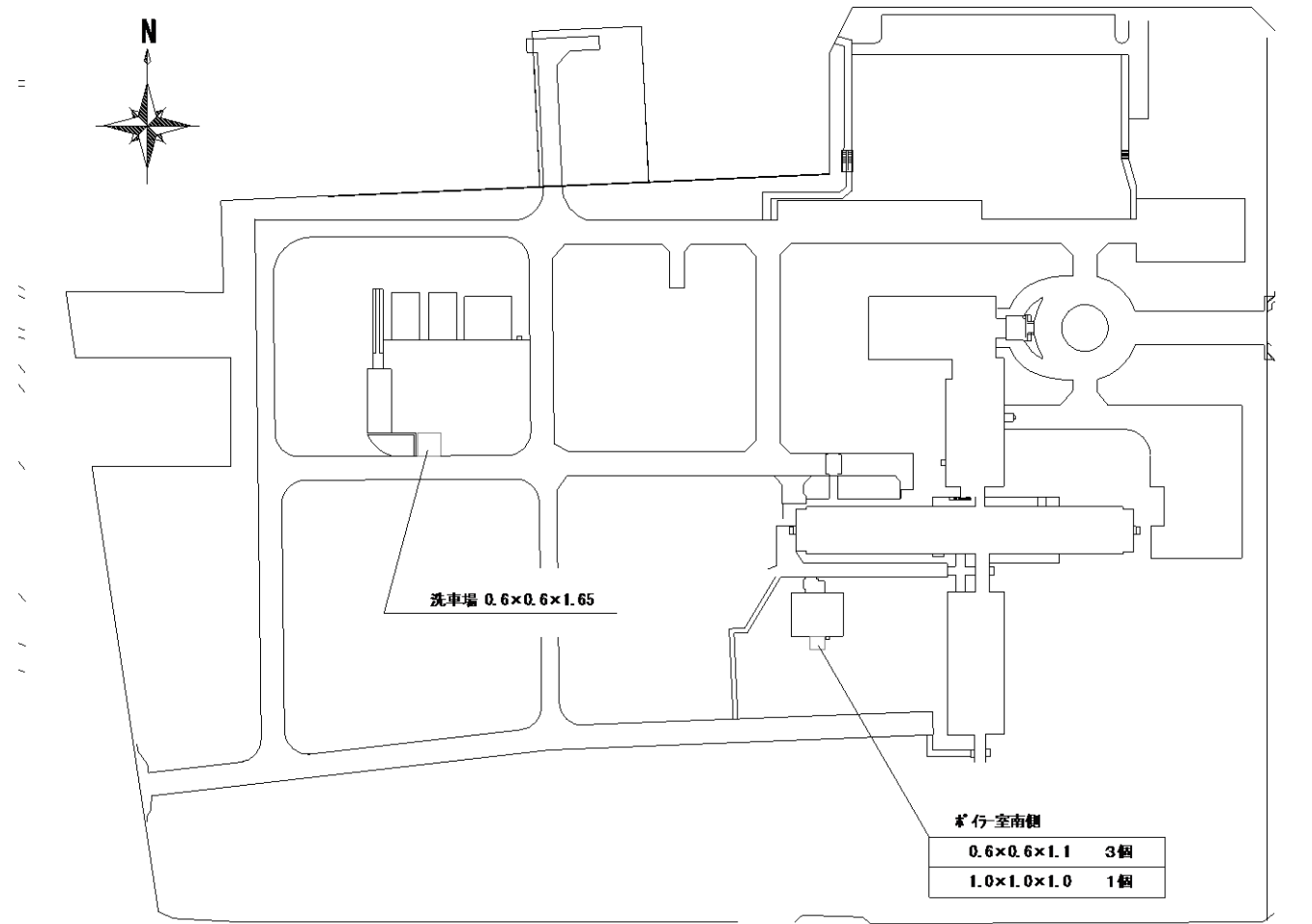
駐屯地配置図 S=1/2,000
