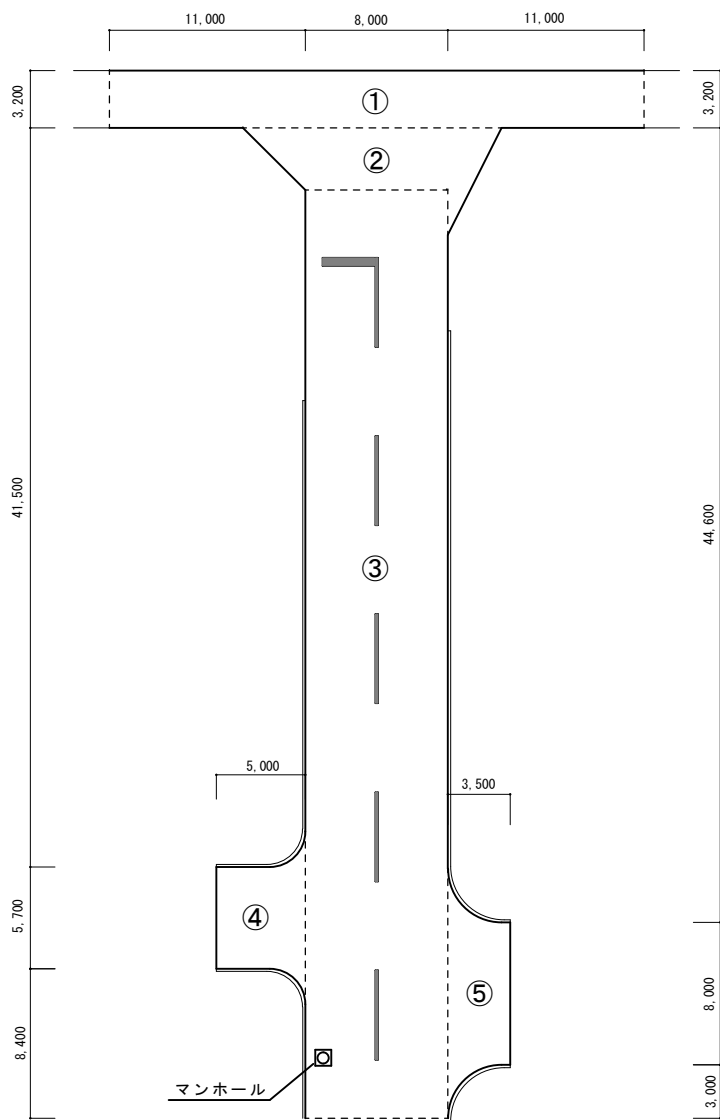
道路工区割平面図 S = 1 / 3 0 0
