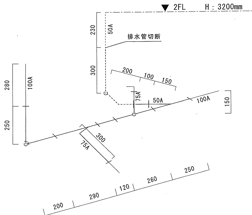
既設排水管図 S = 1/10
