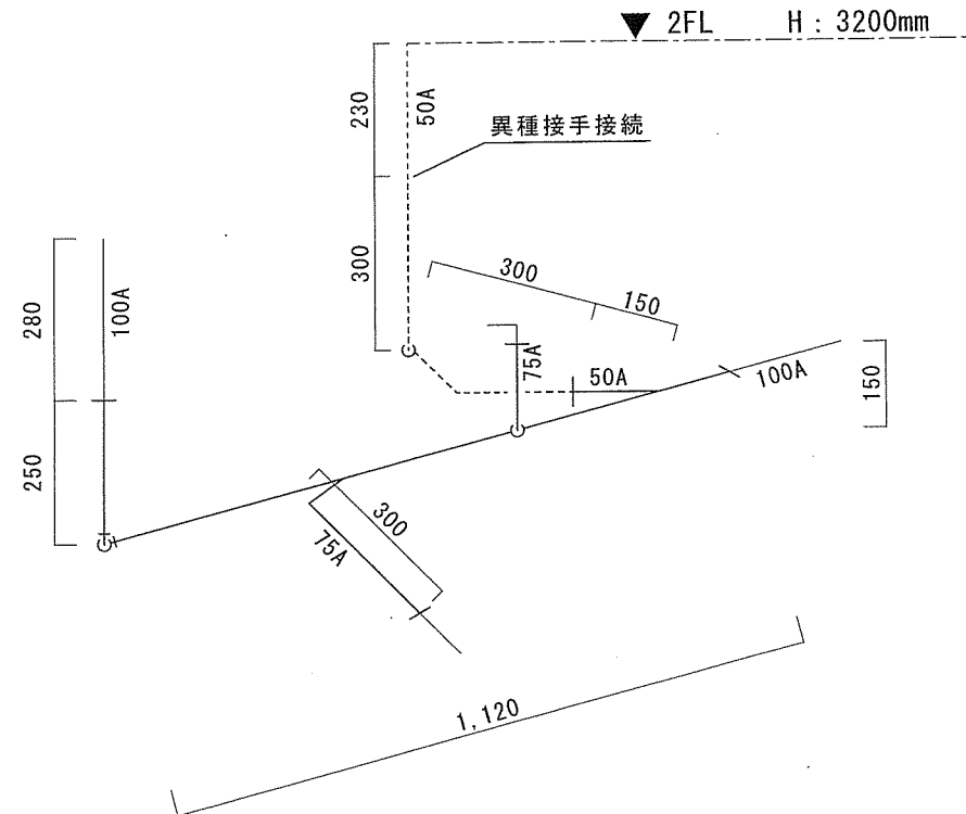
新設排水管図 S = 1 / 1 0
