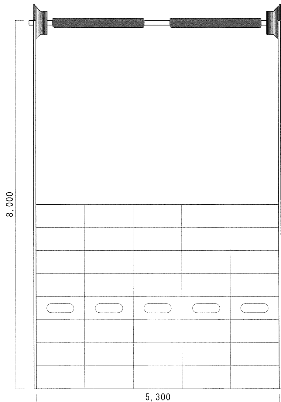
オーバーサイズドア内観図 S=1/50
