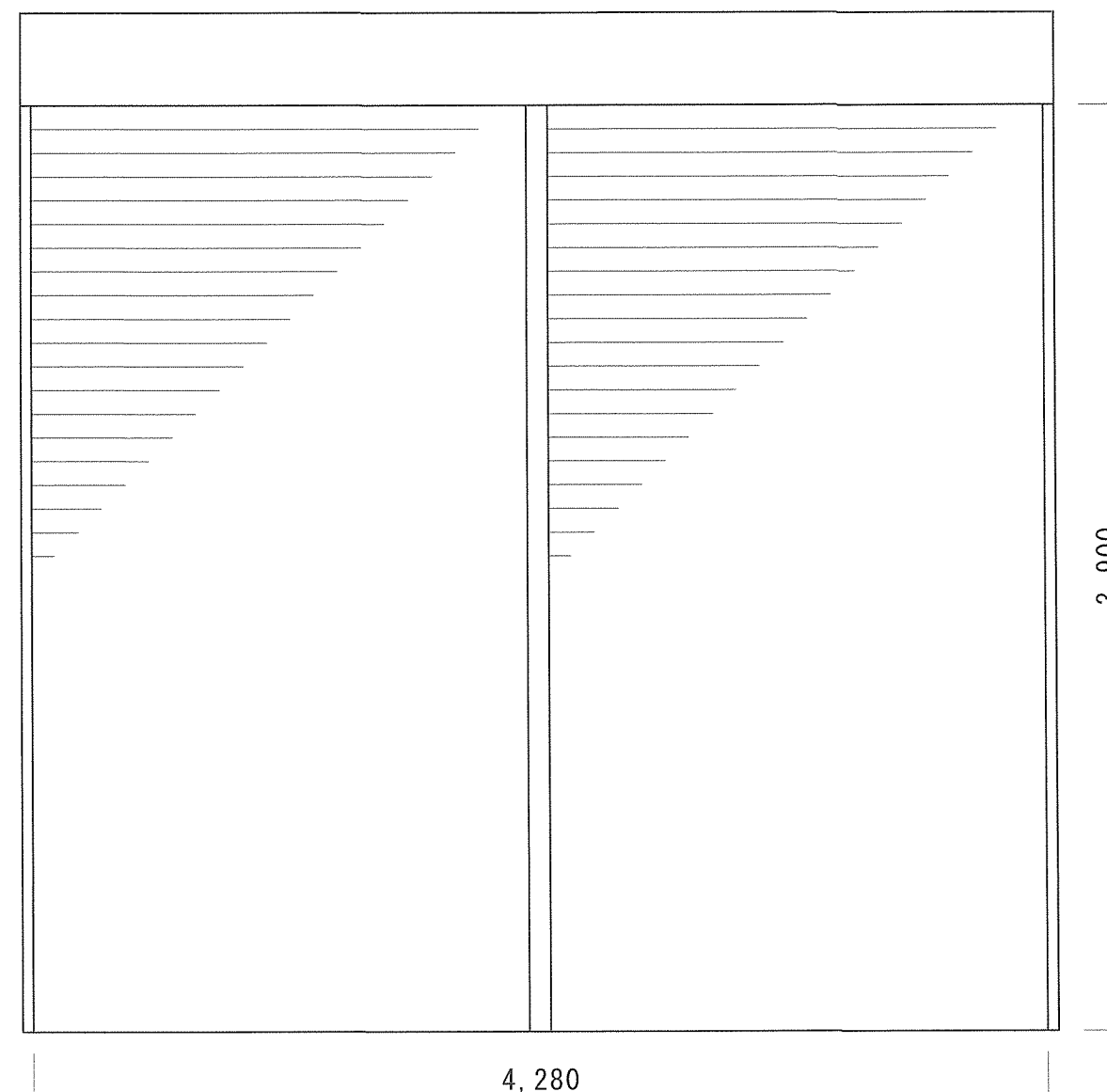
シャッター内観図 S=1/30
