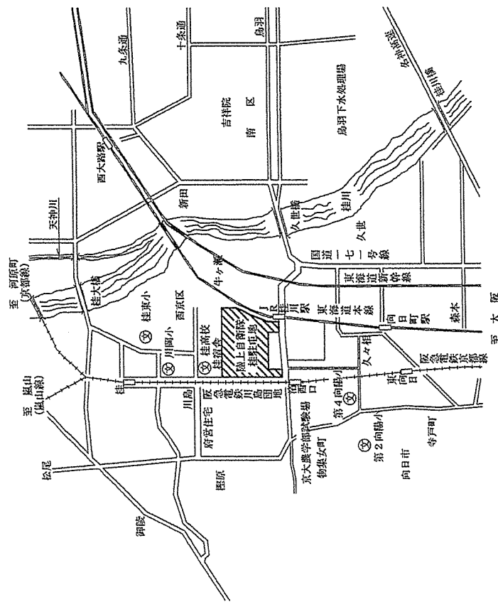
案内図 S=1/40000
