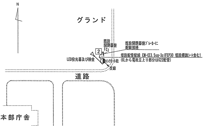
グラント南東投光器柱 工事図 S=1/1000
