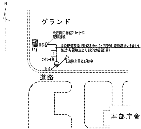
グラント南西投光器柱 工事図 S=1/1000
