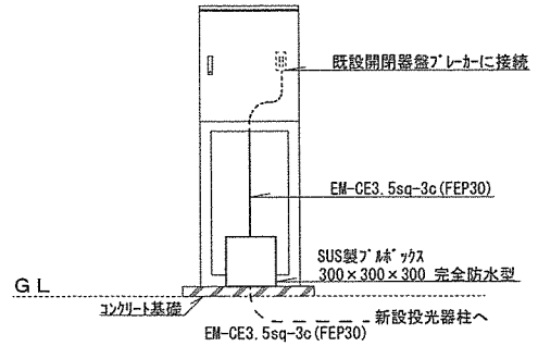
既設開閉器盤 詳細図 1/50
