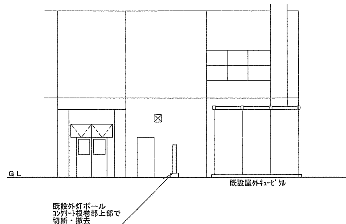
工事箇所②詳細図(補修前) S=1/200
