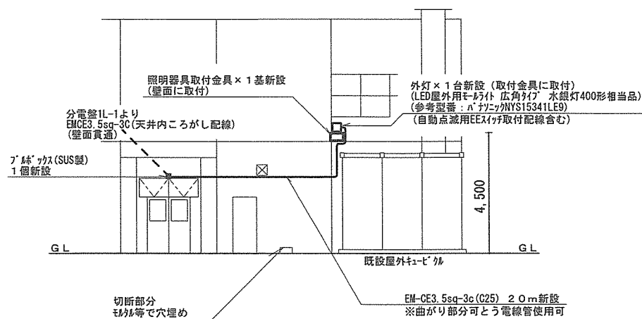
工事箇所②詳細図(補修後) S=1/200
