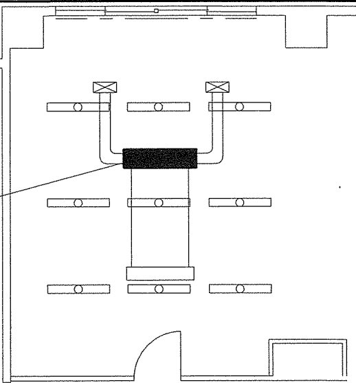
工事場所A拡大図 S=1/100
