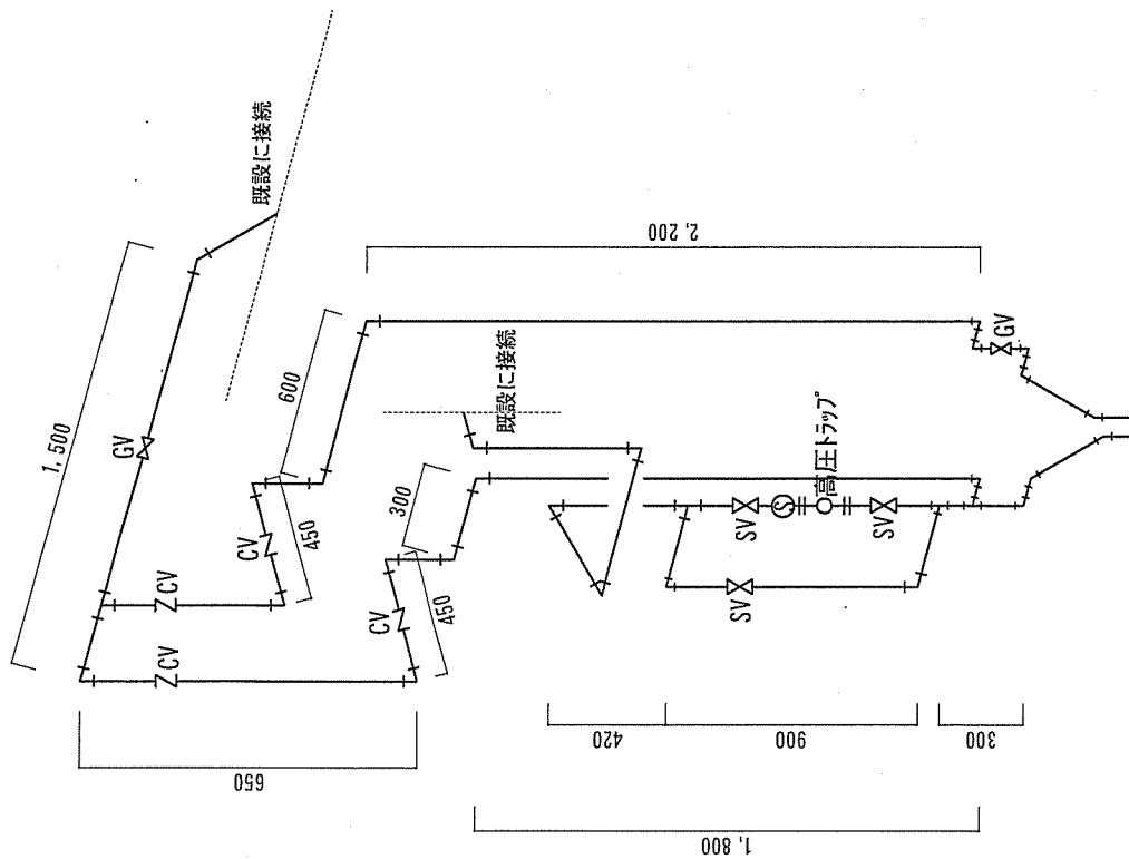
食厨トラップ廻り配管系統図
