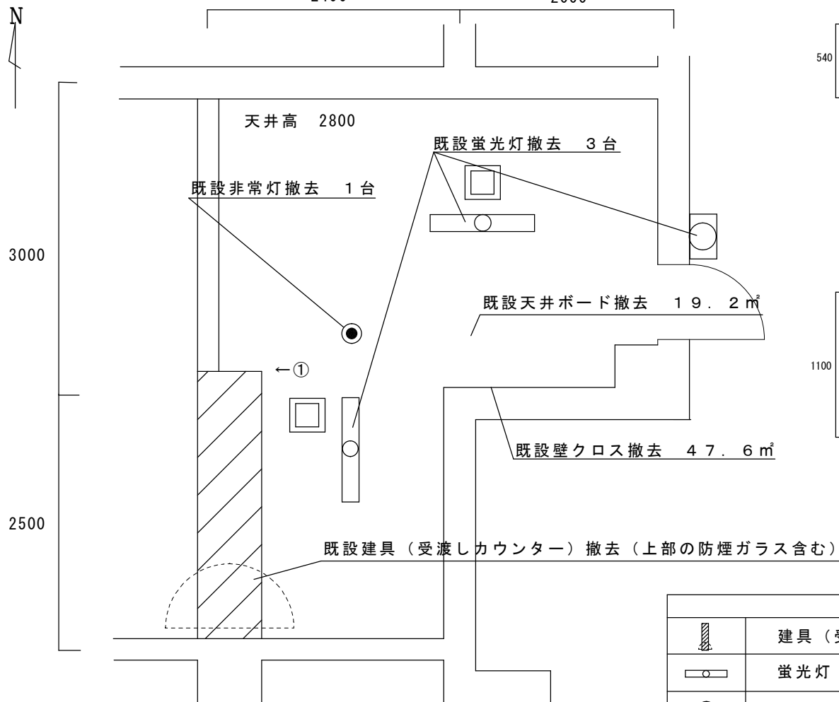
撤去平面図 S = 1 / 8 0 0
