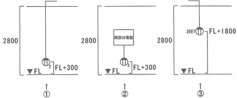
新設展開図② S = N S
