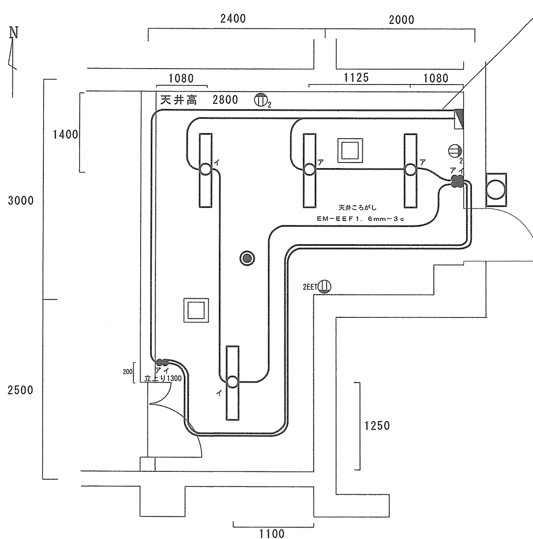
新設平面図③ S=1/800
