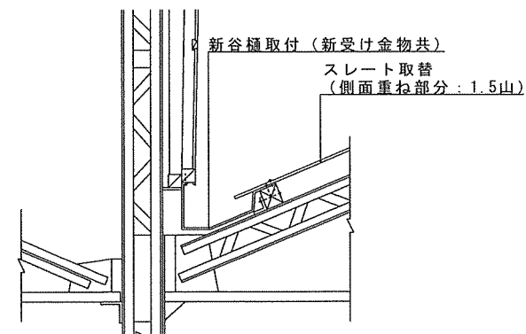
新雨樋標準断面図
