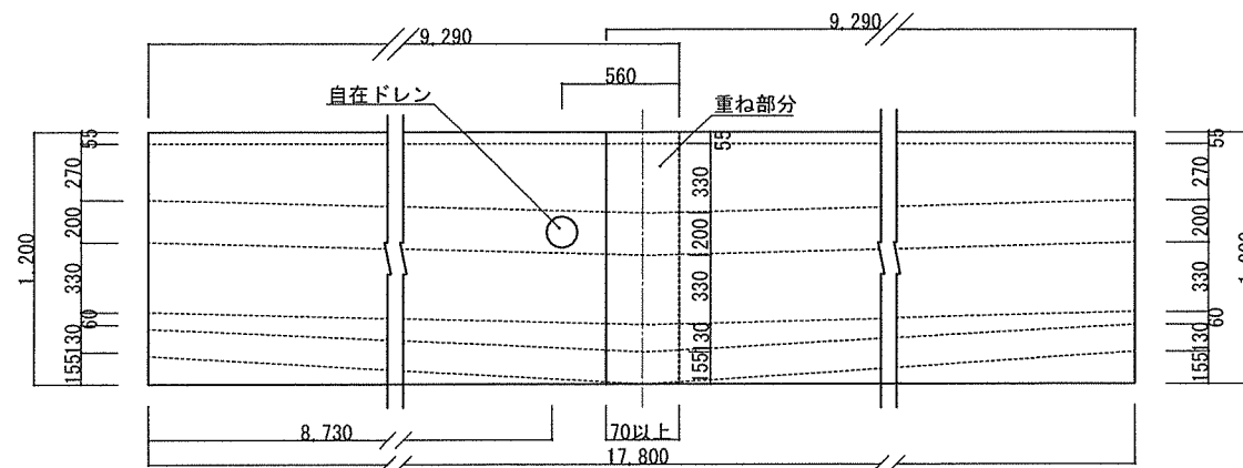
谷とい正面図 S=1/40
