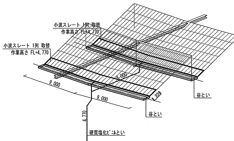
雨とい補修標準図
