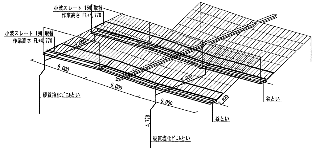
雨とい補修標準図
