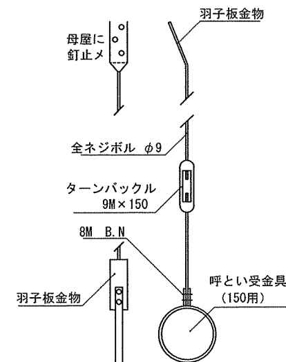
呼とい受金具詳細図
