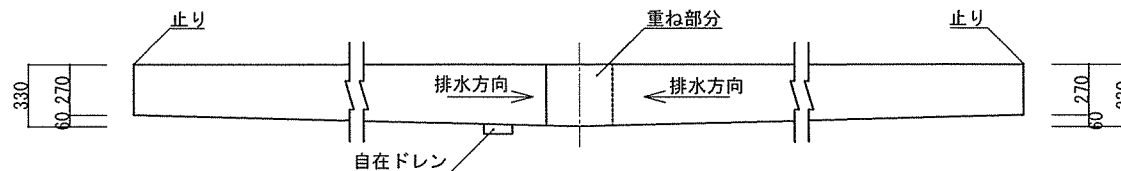
谷とい正面図 S=1/40
