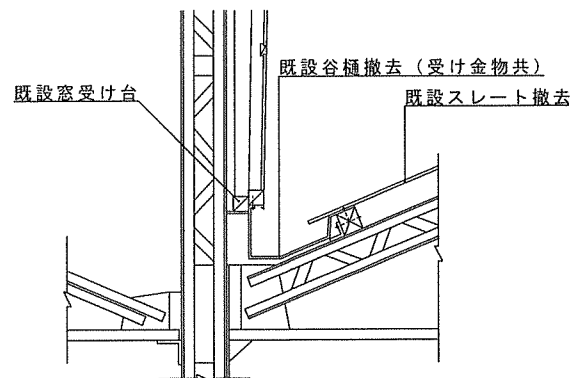
既設雨樋標準断面図
