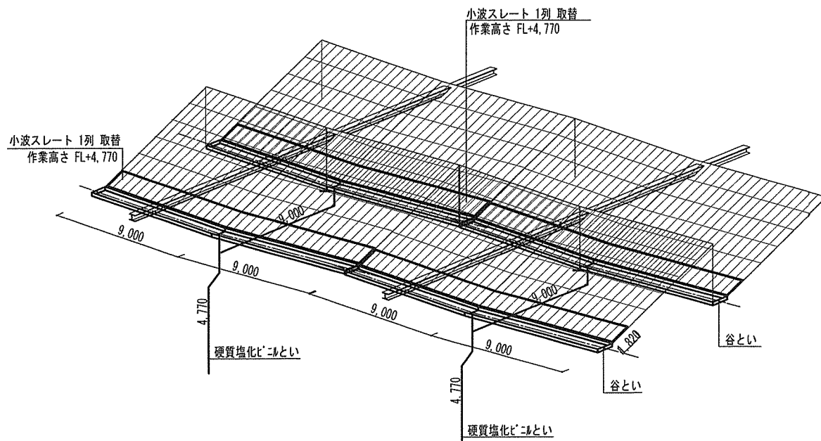
雨とい補修標準図
