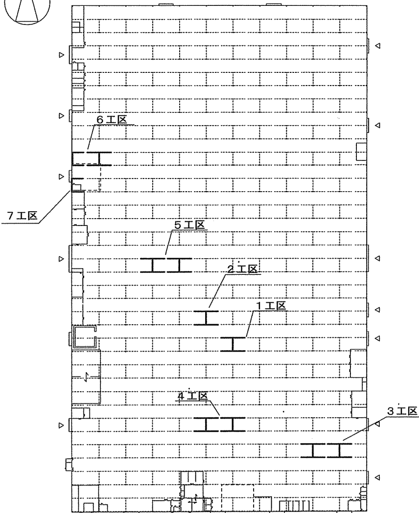
17号建物平面図 S=1/2500
