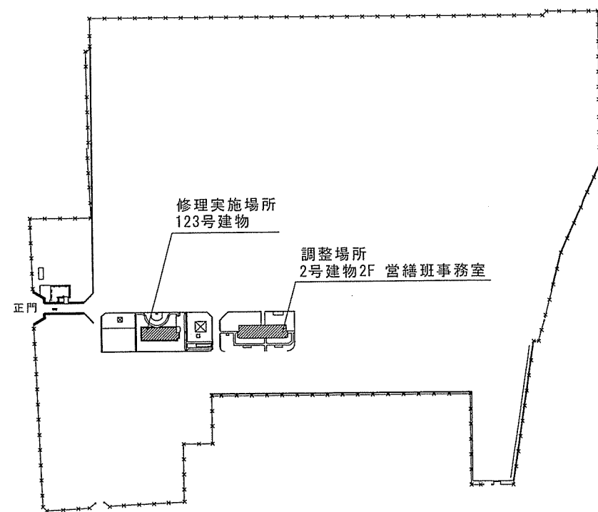
配置図 S=1/5,000
