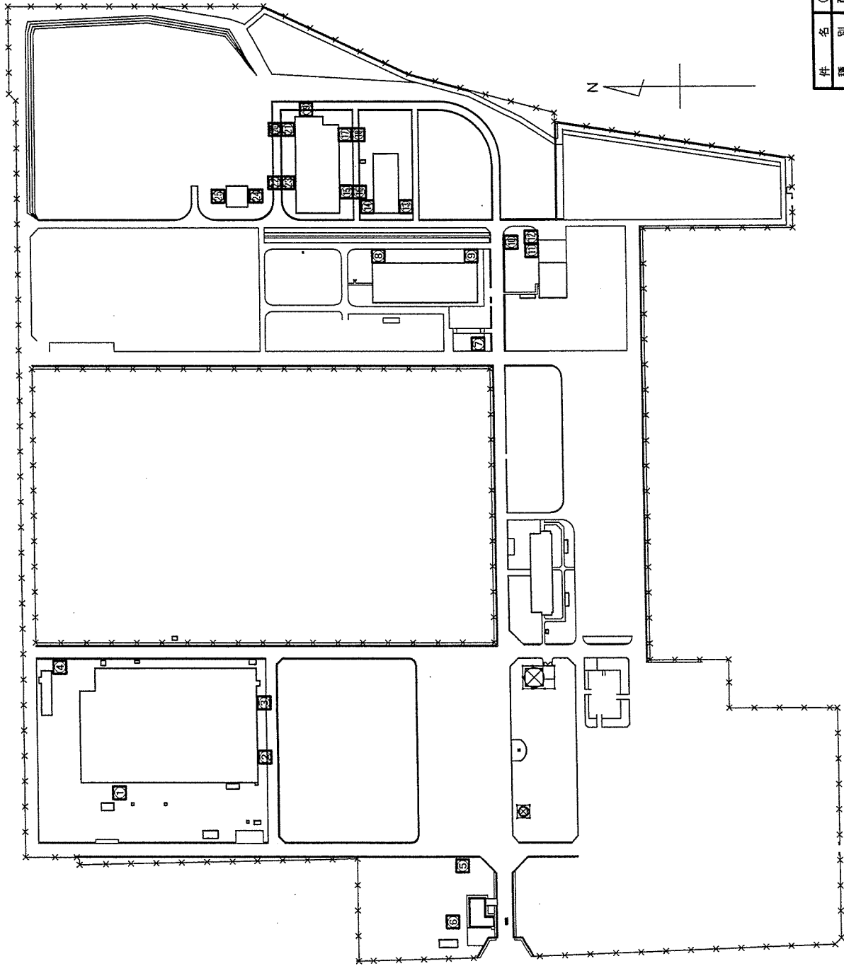
(6) 油分離槽配置圖
