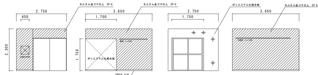
洋室A壁展開図 S=1/100
