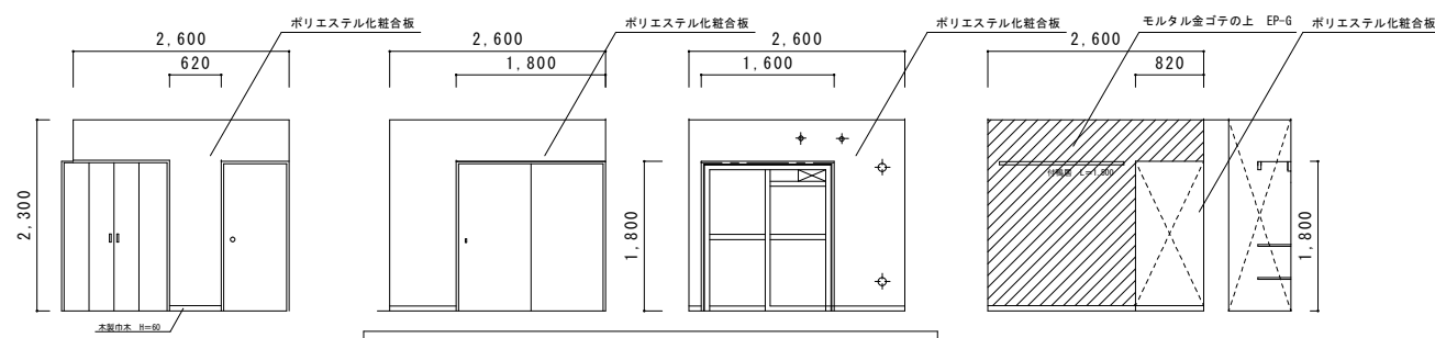
洋室B壁展開図 S=1/100
