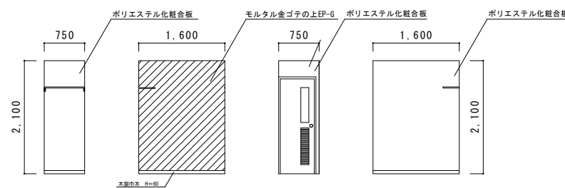
便所壁展開図 S=1/100
