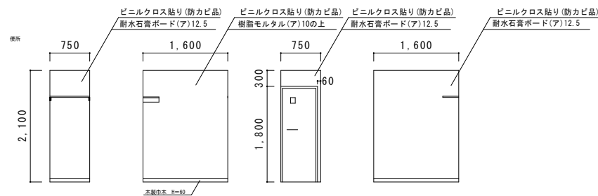
便所壁展開図 S=1/100
