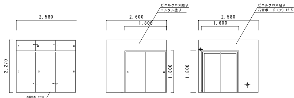
洋室 B 壁展開図 S=1/100
