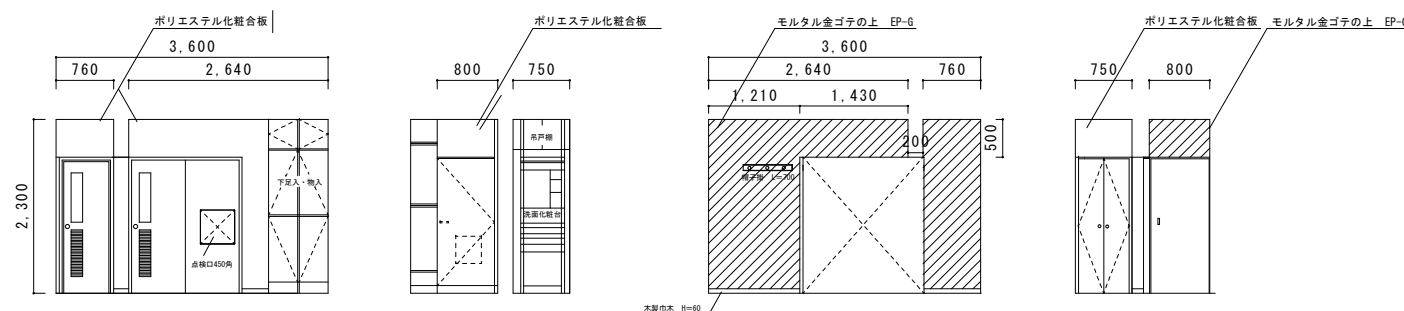
玄関・ホール壁展開図 S=1/100
