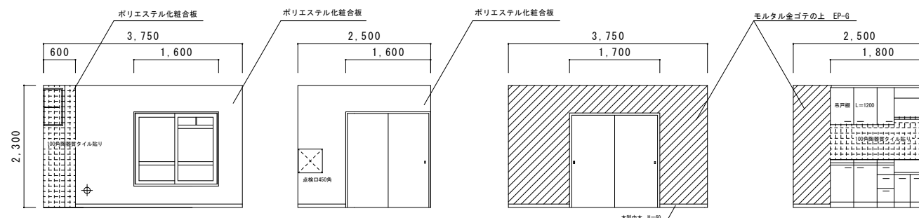
台所・食事室壁展開図 S=1/100
