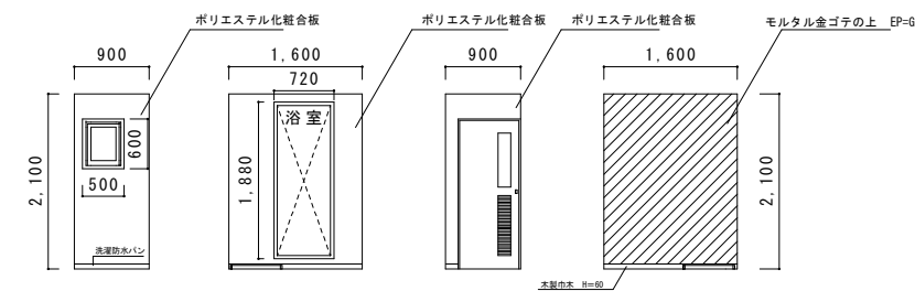
洗濯室壁展開図 S=1/100
