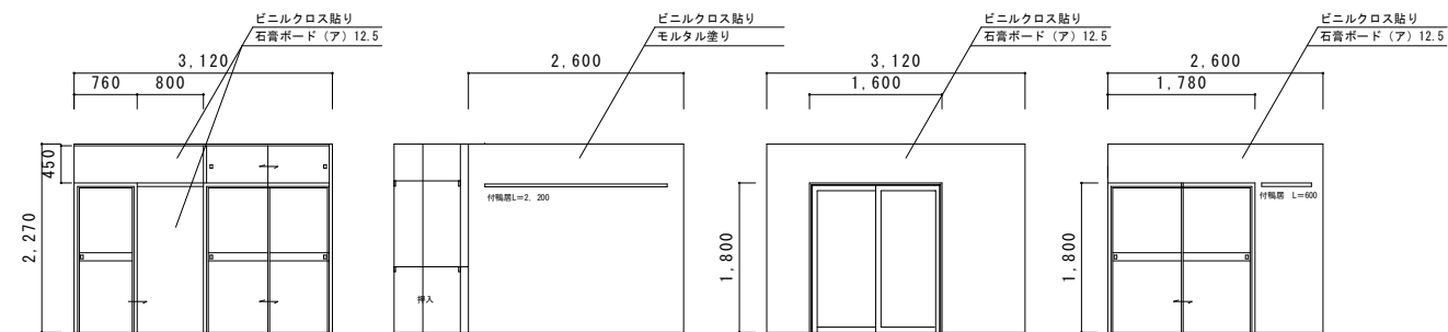
和室壁展開図 S=1/100
