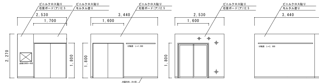
台所・食事室壁展開図 S=1/100
