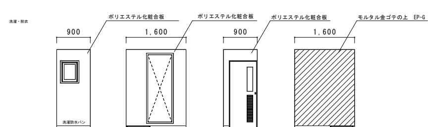
洗濯室壁展開図 S=1/100
